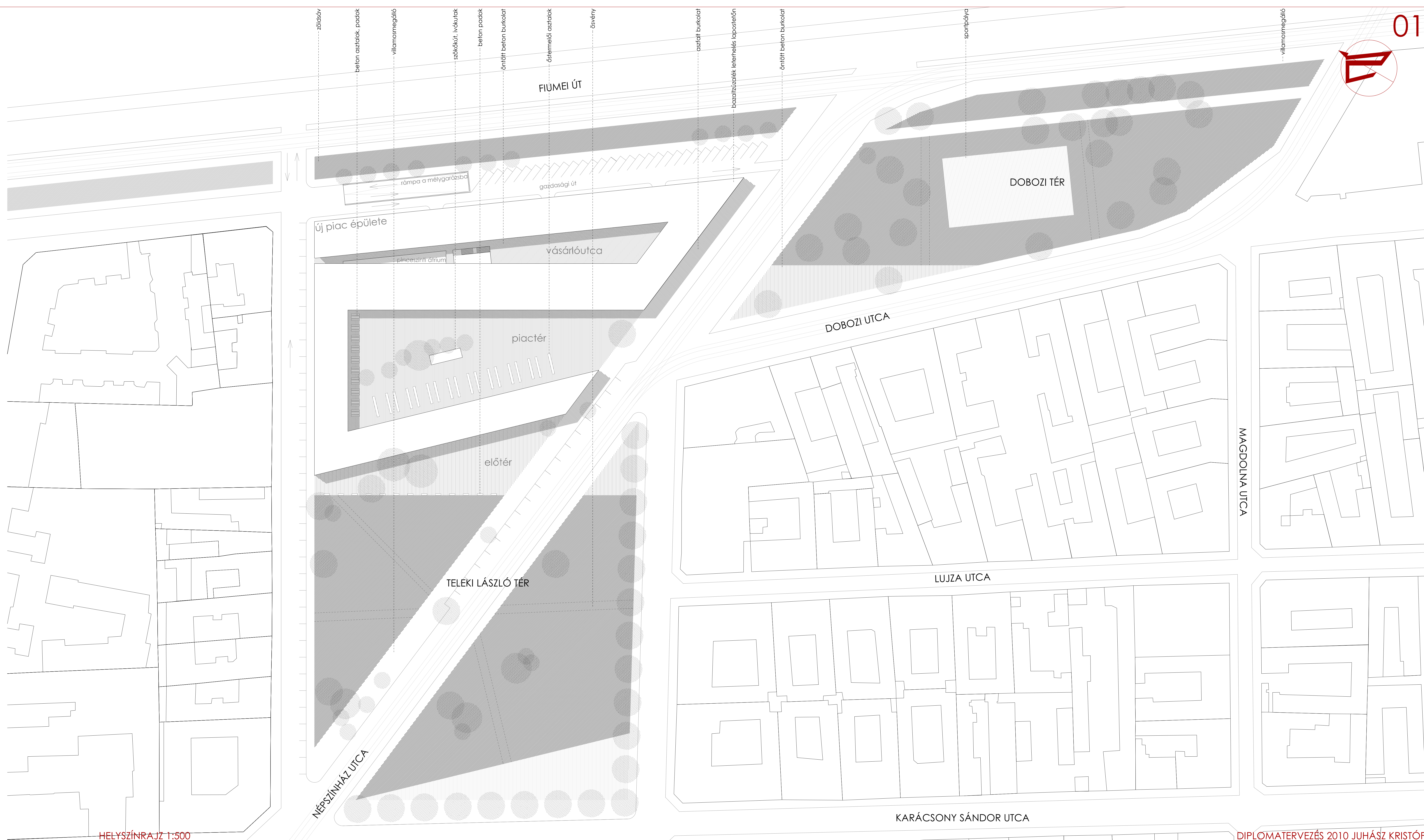
HELYSZÍNRAJZ 1:500
