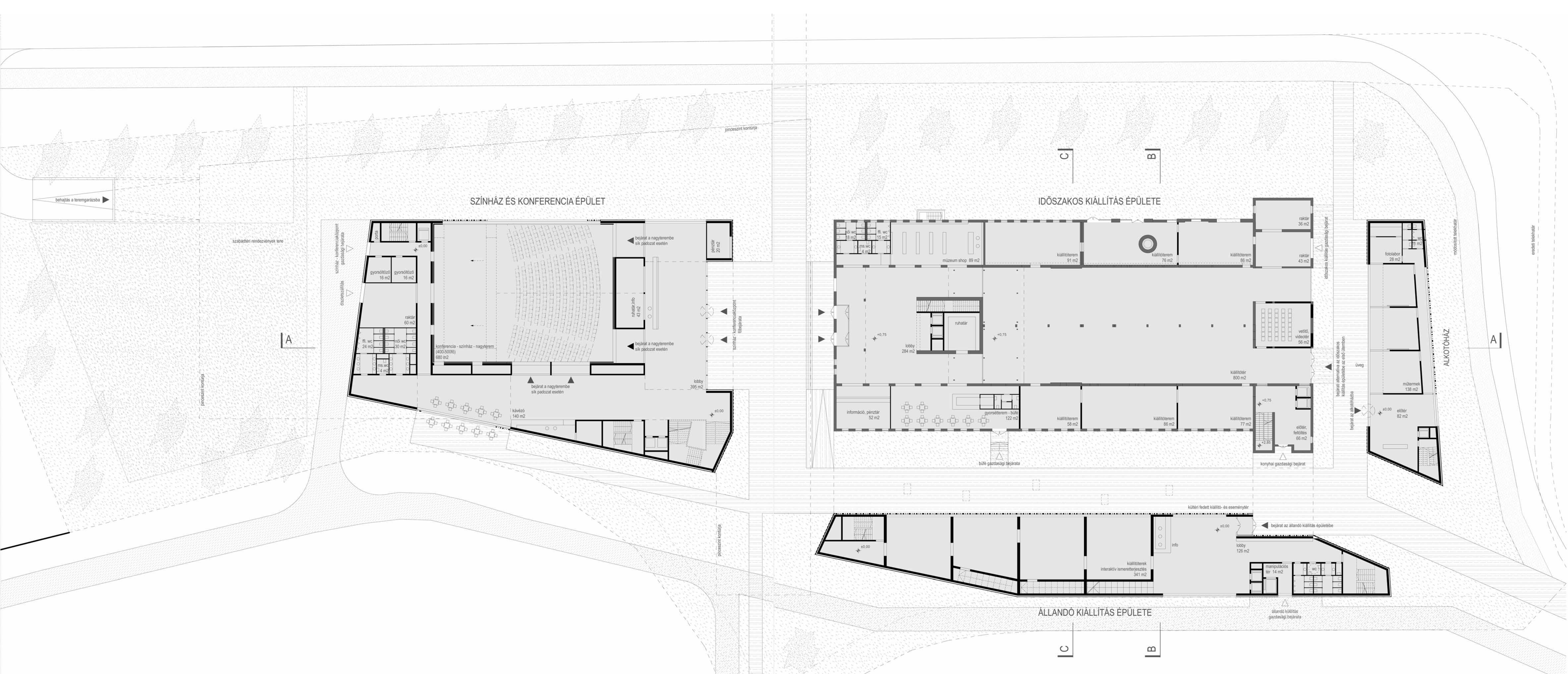
FÖLDSZINTI ALAPRAJZ
