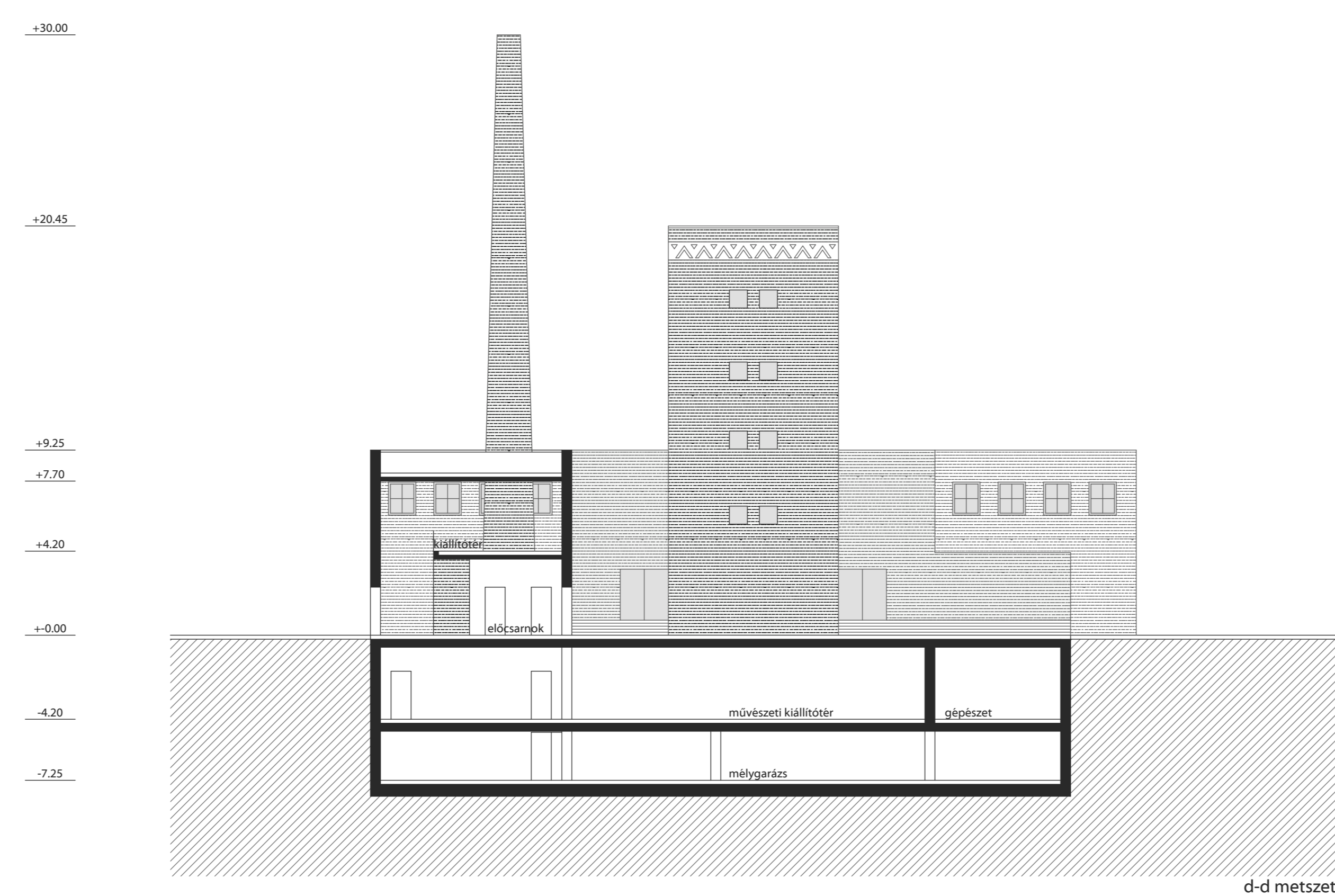
d-d metszet
