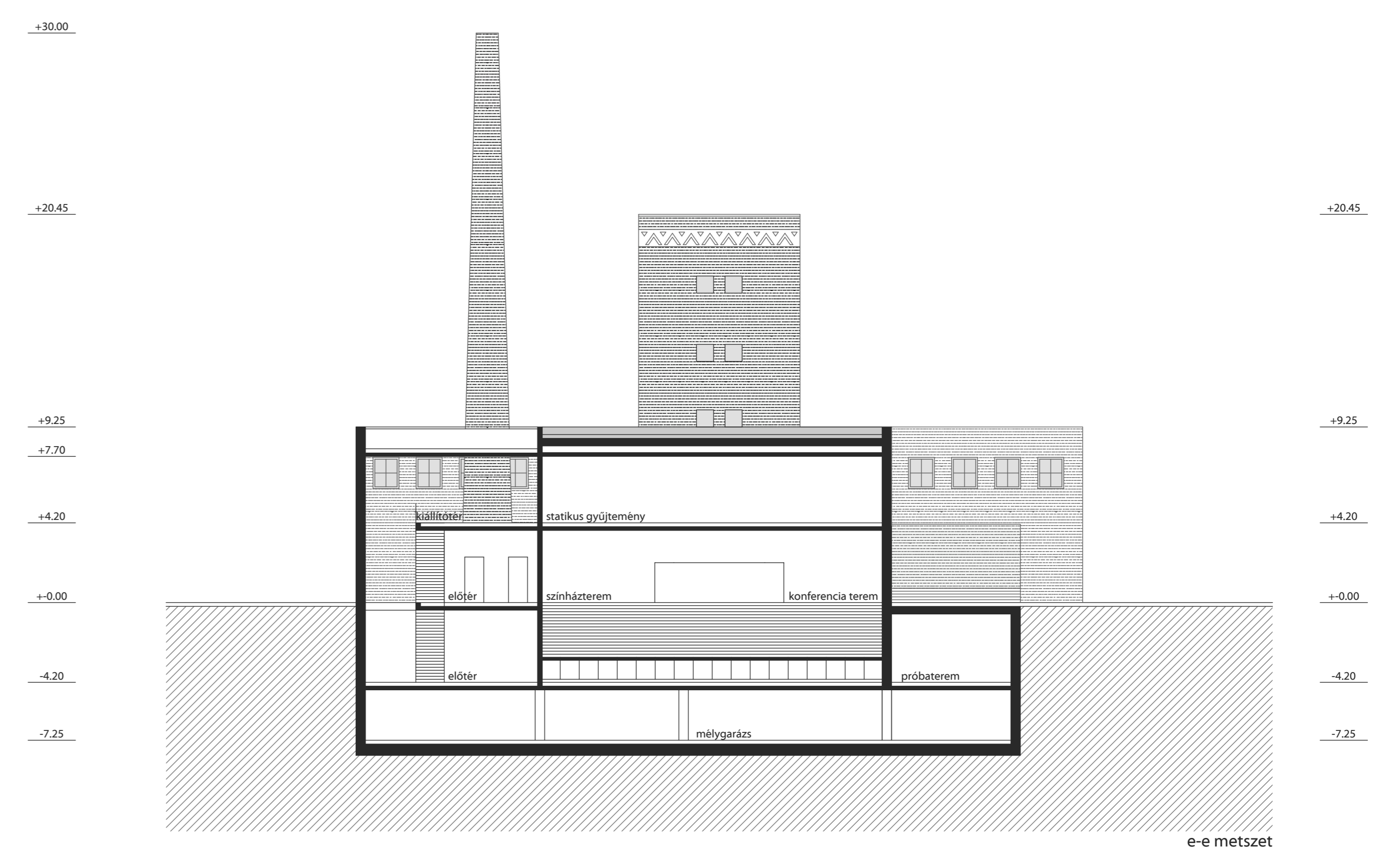
e-e metszet
