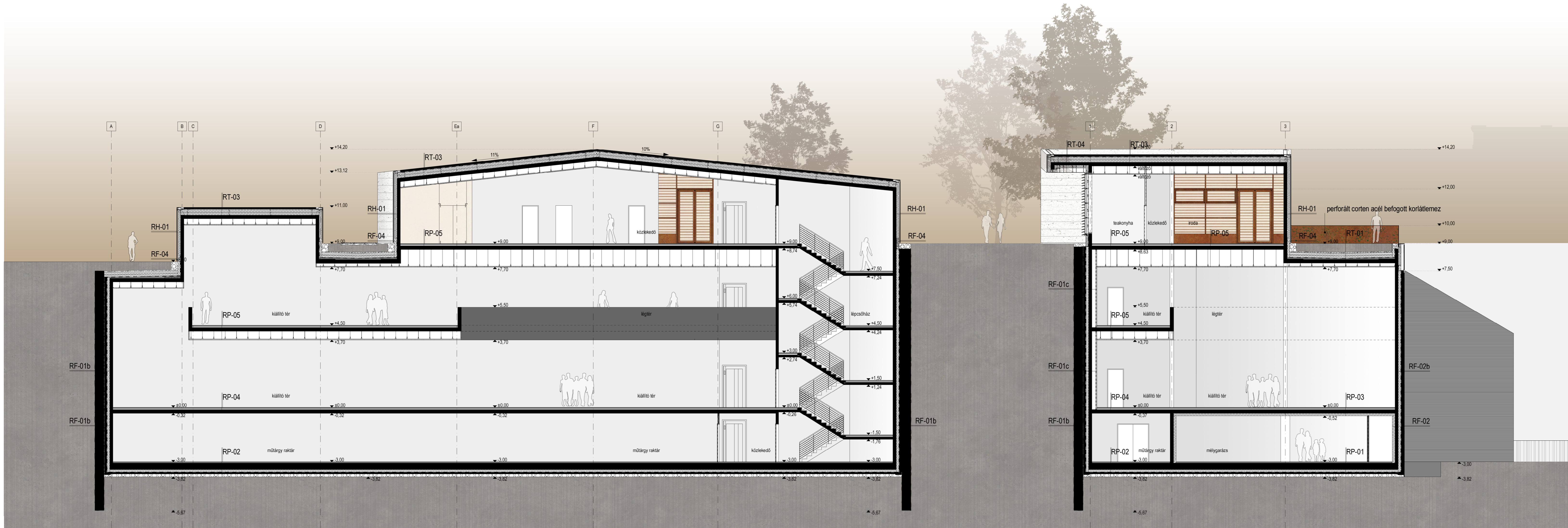
B-B METSZET E-E METSZET M=1:100
