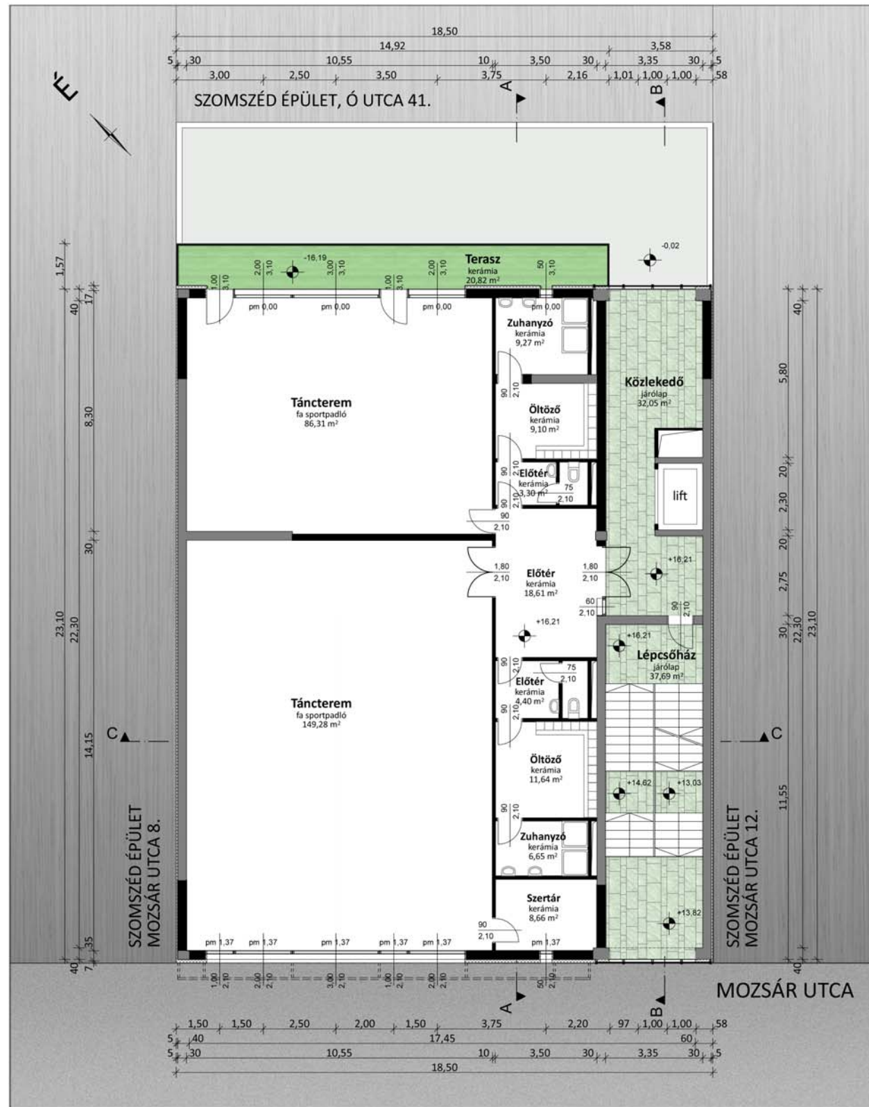
3. EMELET ALAPRAJZA M=1:100
