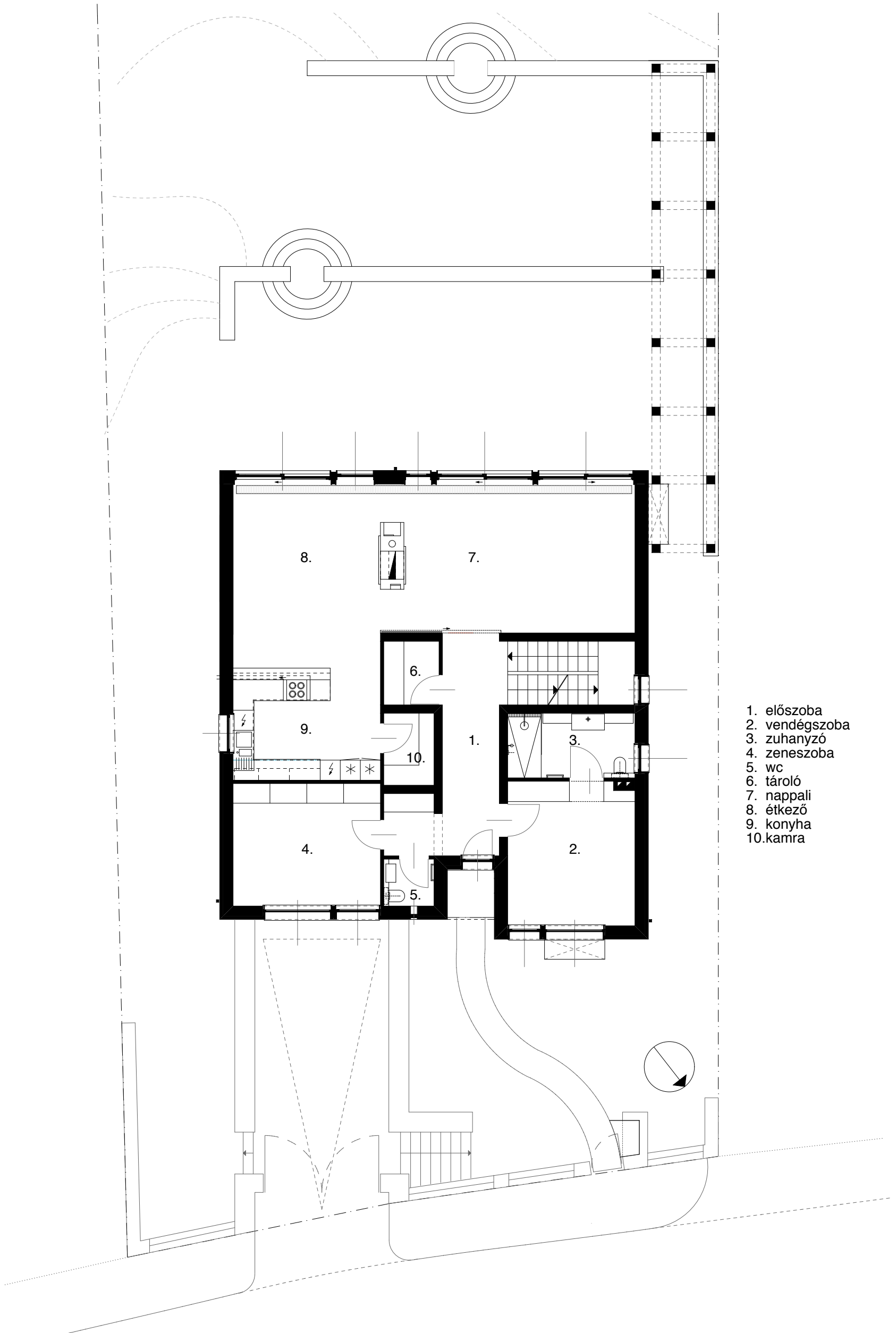
FÖLDSZINTI ALAPRAJZ
