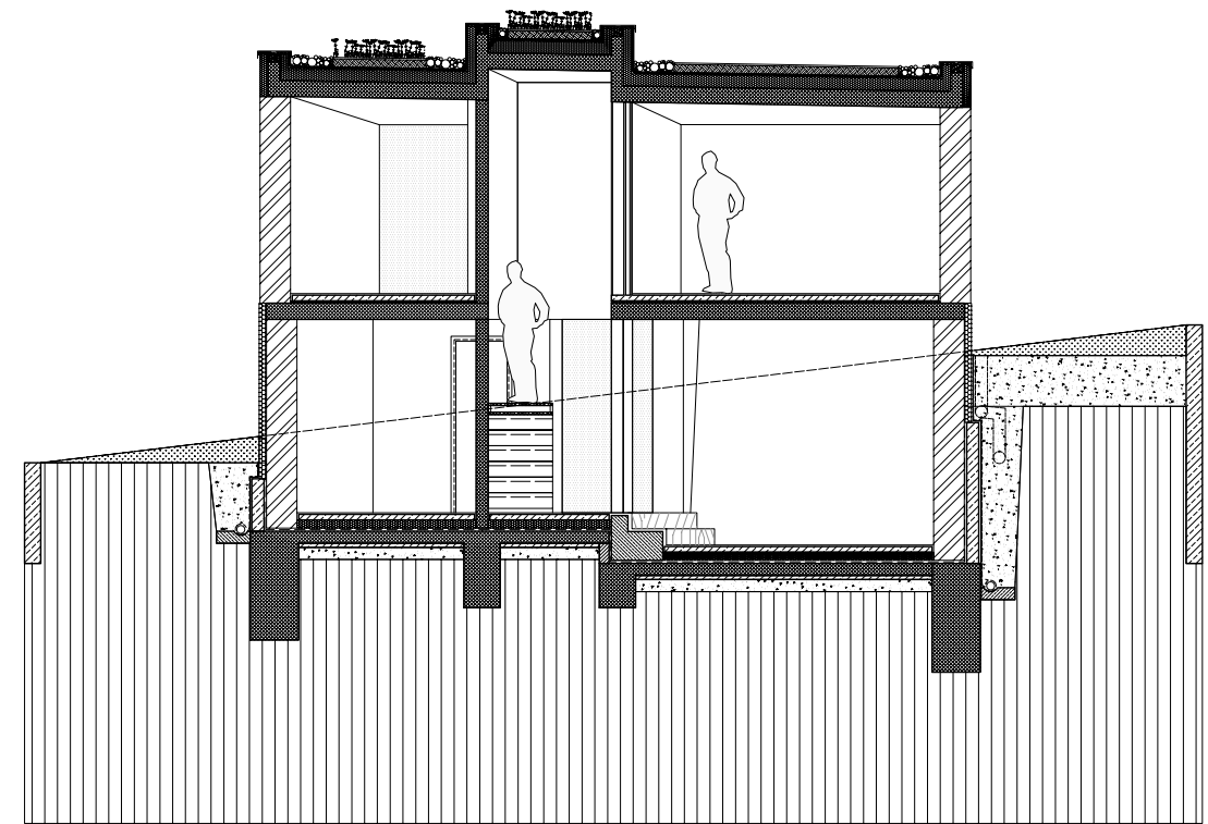
BALATONAKARATTYAI NYARALÓ KERESZTMETSZET
