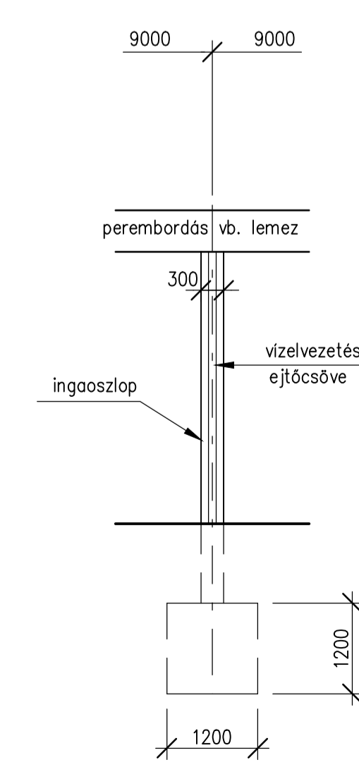
KERESZTMETSZET
