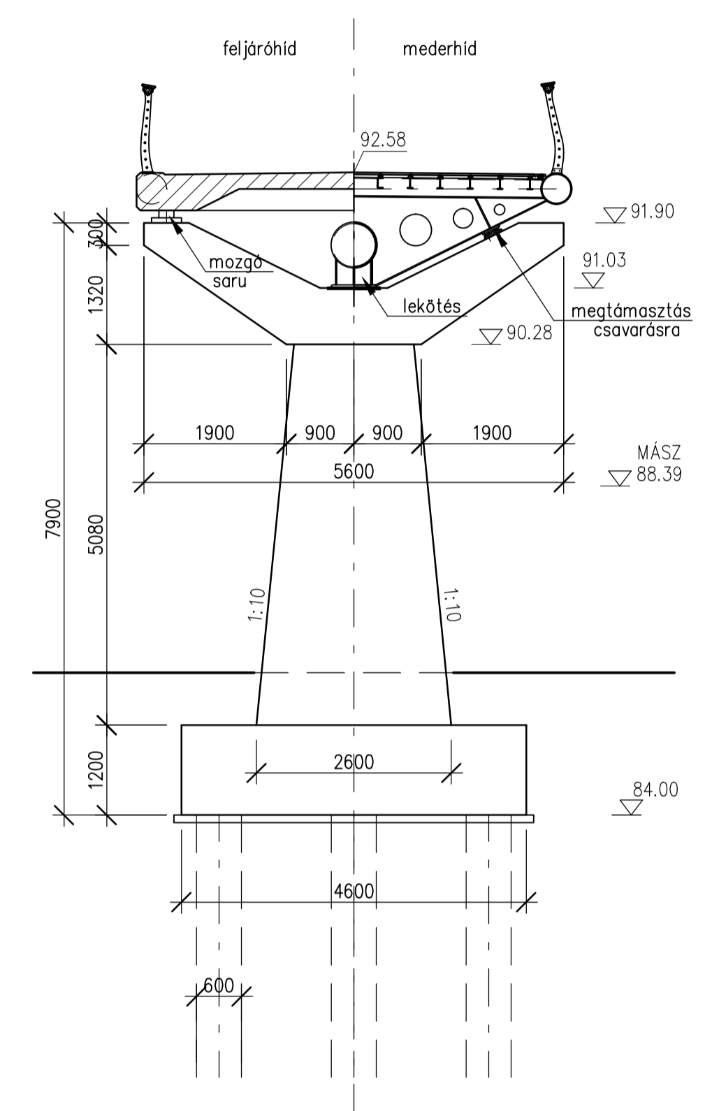
KERESZTMETSZET
