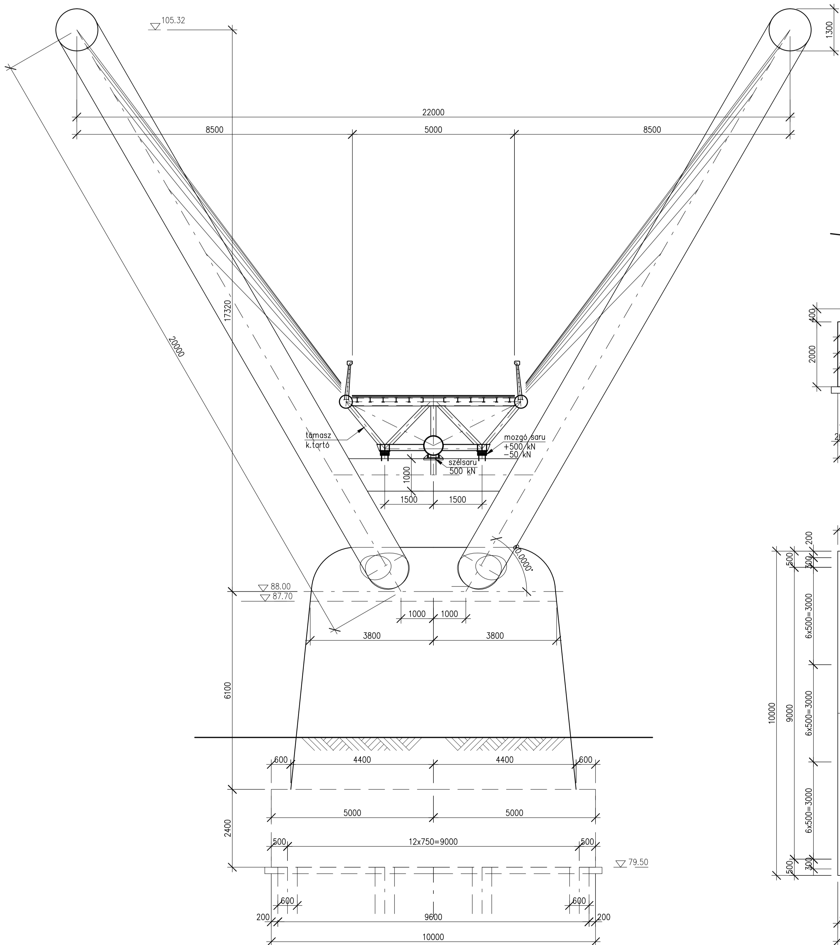
KERESZTMETSZET
