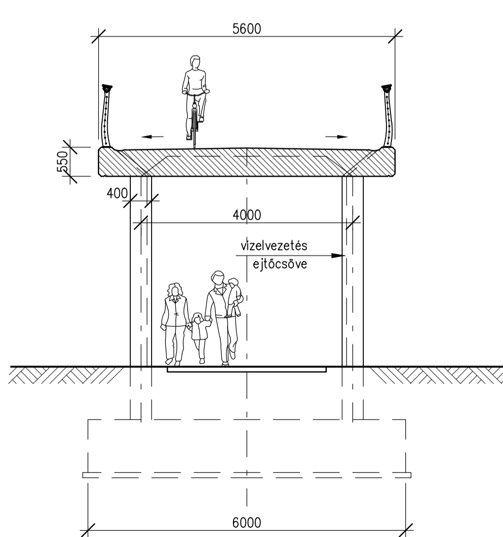
HOSSZMETSZET
