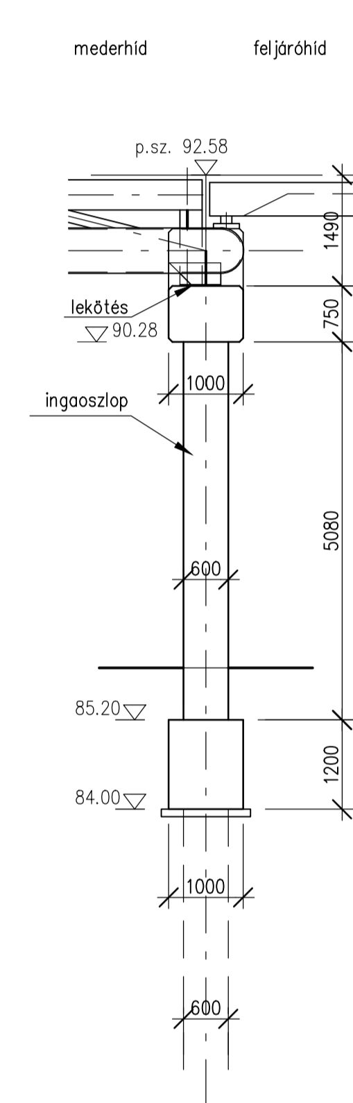
HOSSZMETSZET
