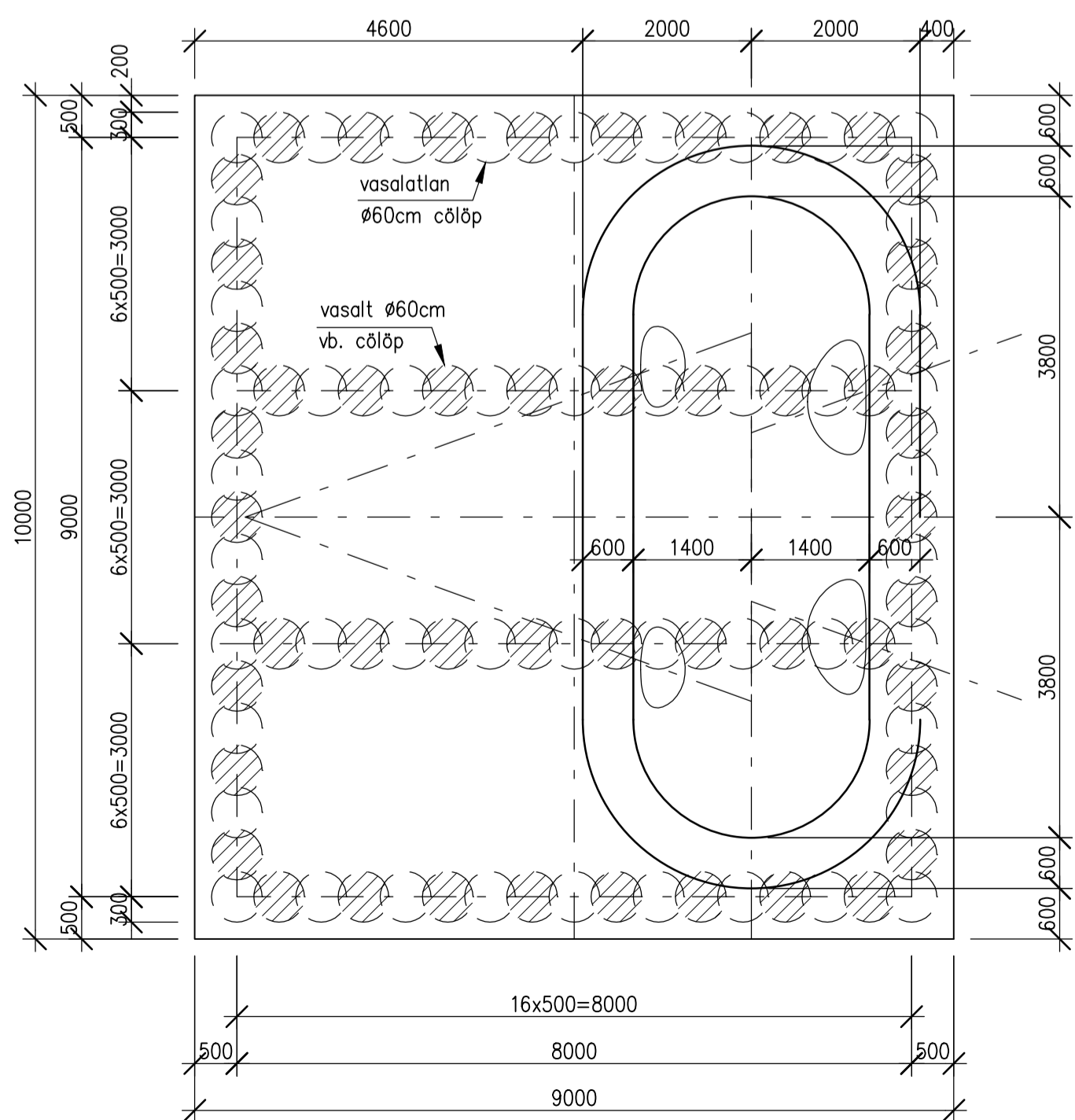
FELÜLNÉZET
