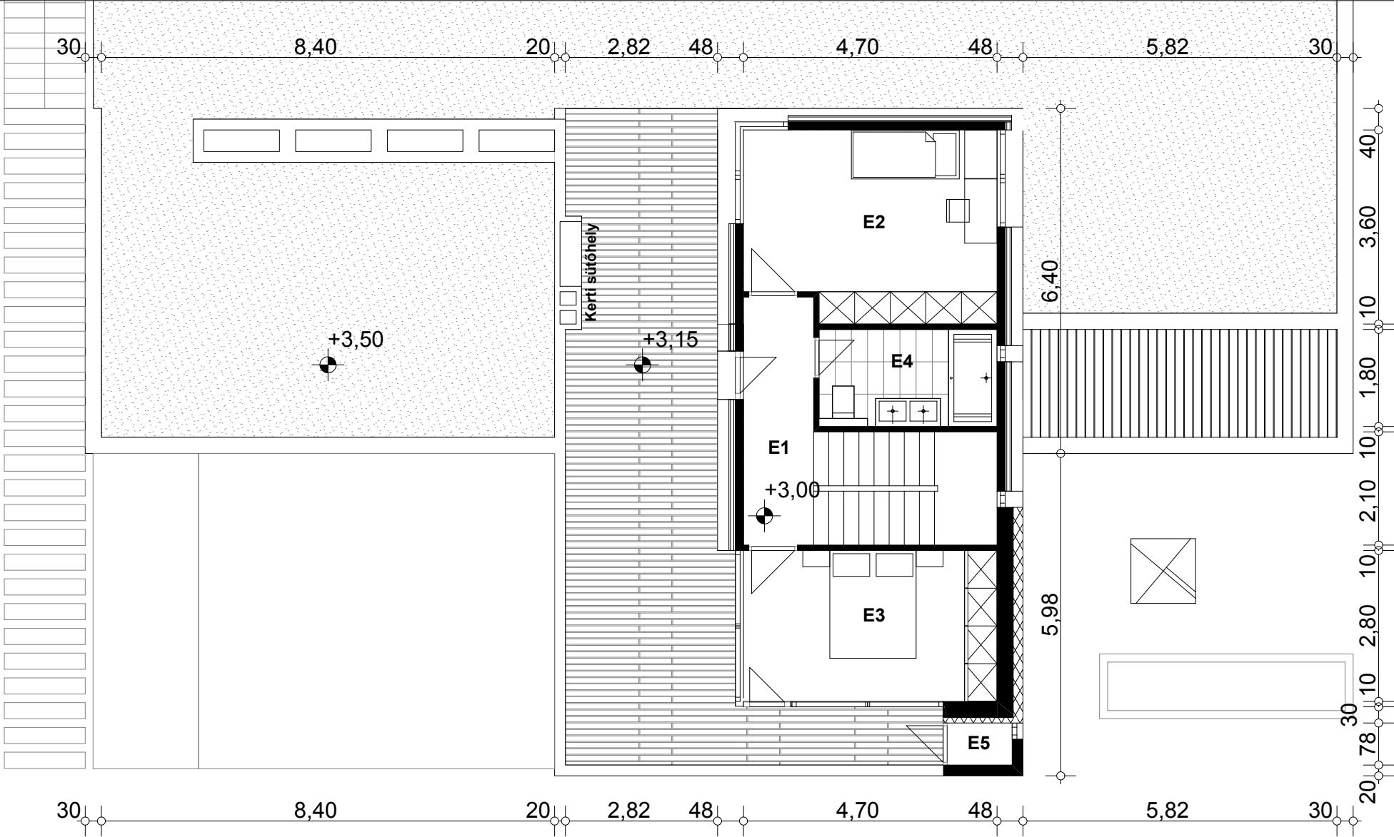
EMELETI ALAPRAJZ M 1:100
