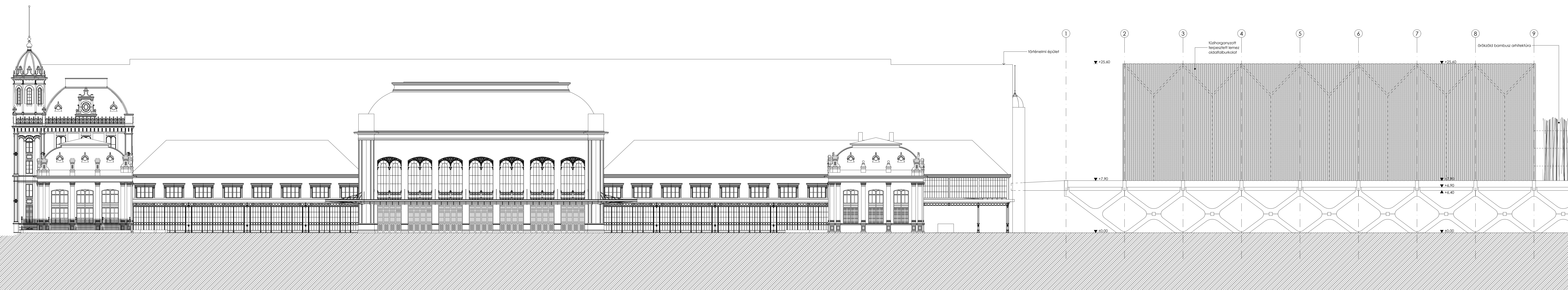
DÉL-KELETI HOMLOKZAT RÉSZLET I.
