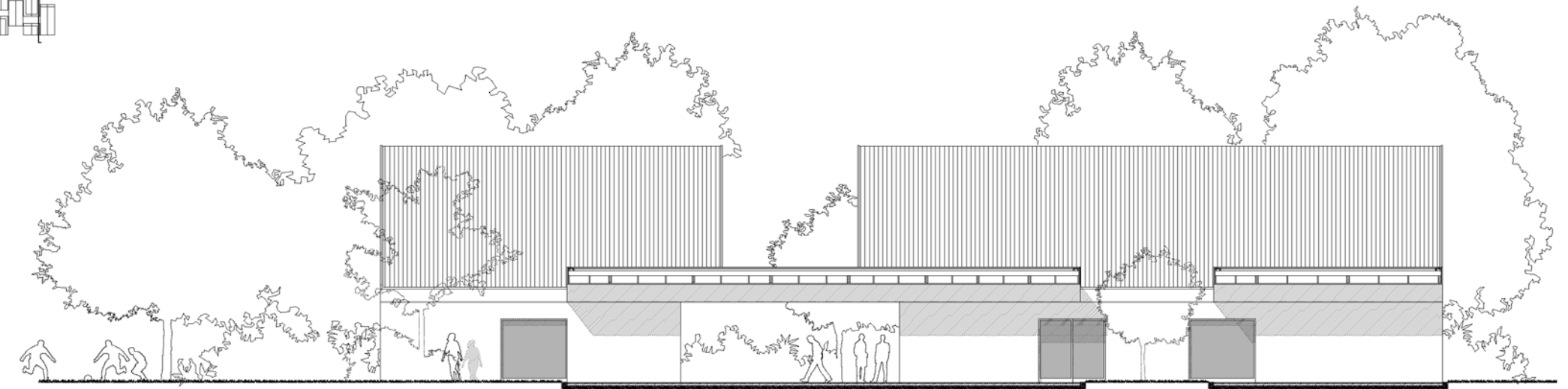
II METSZET
