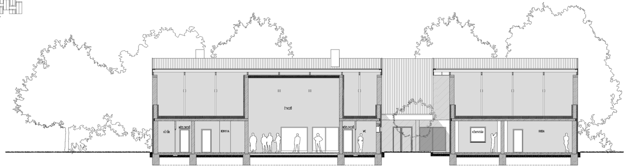
GG METSZET
