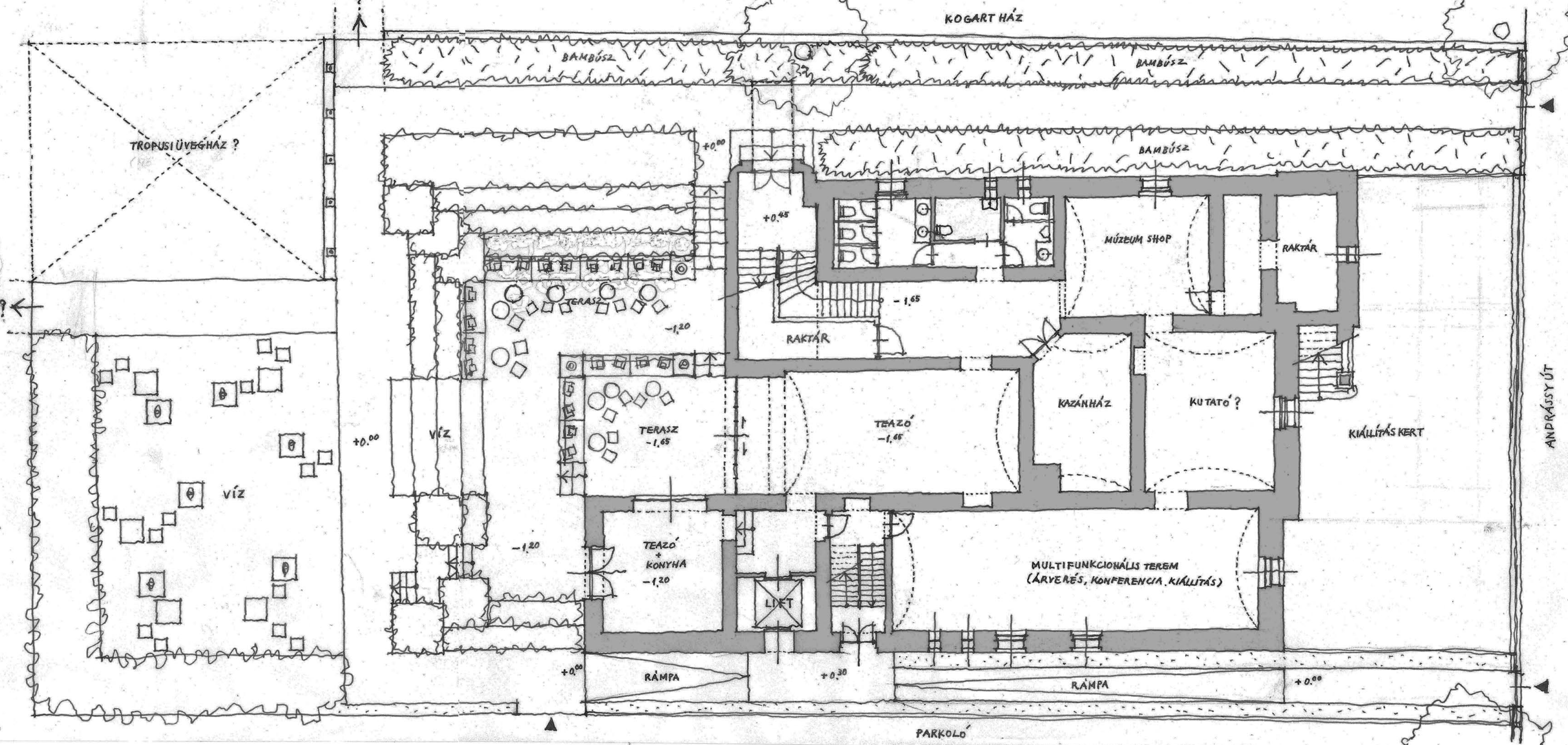
DK Ázsia Múzeum - alagsor tervezett alaprajza
