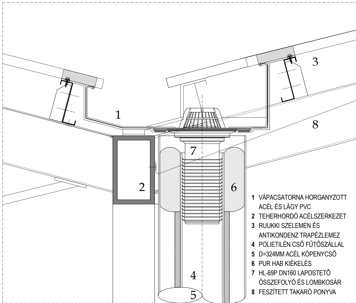
PIACTETŐK VÁPA ÉS ÖSSZFOLYÓ-EJTŐ SZERKEZETI RÉSZLET AZ ELEKTROMOS KÁBELEZÉS, ÉS A VENDÉGLÁTÓ HELY KÉMÉNYE IS OSZLOPON KERESZTÜL VAN FELVEZETVE
