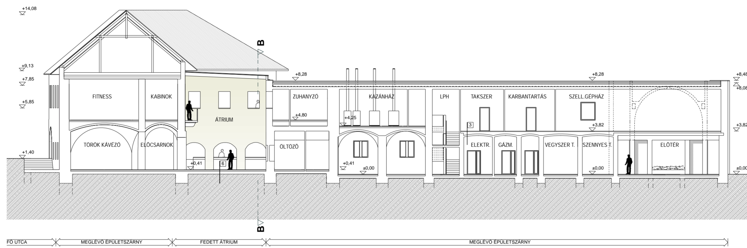
A-A METSZET
