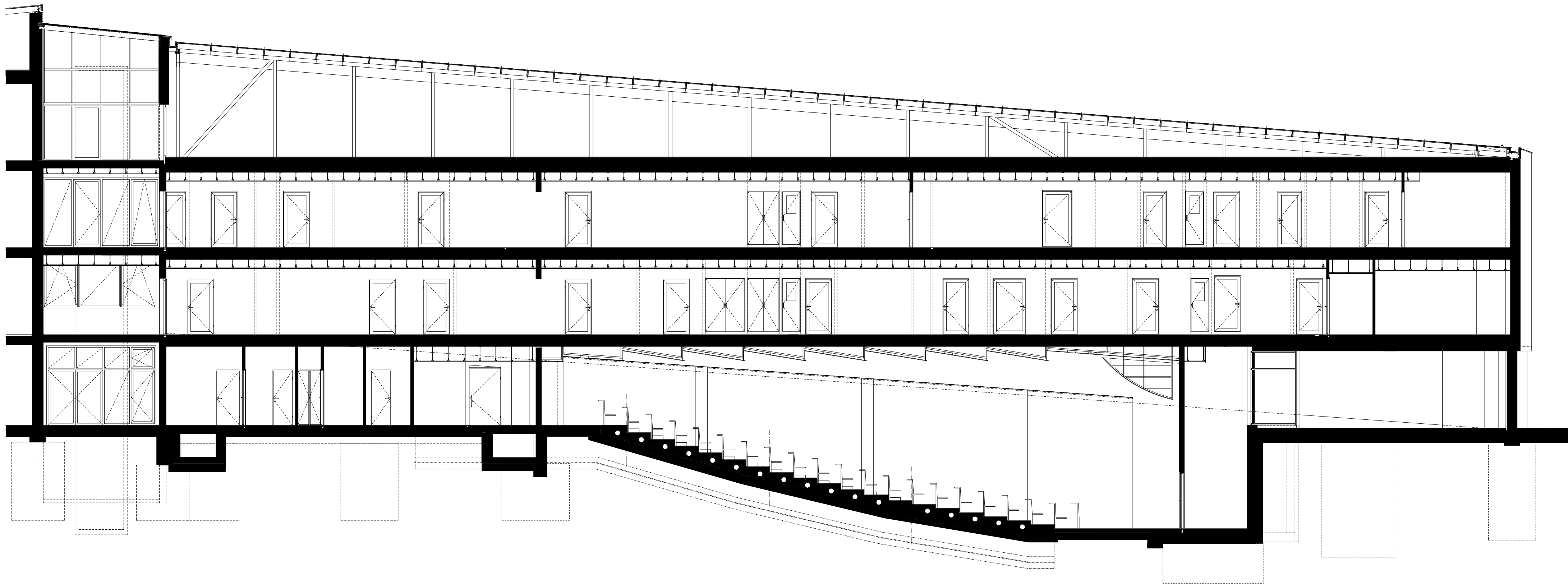
D-D METSZET
