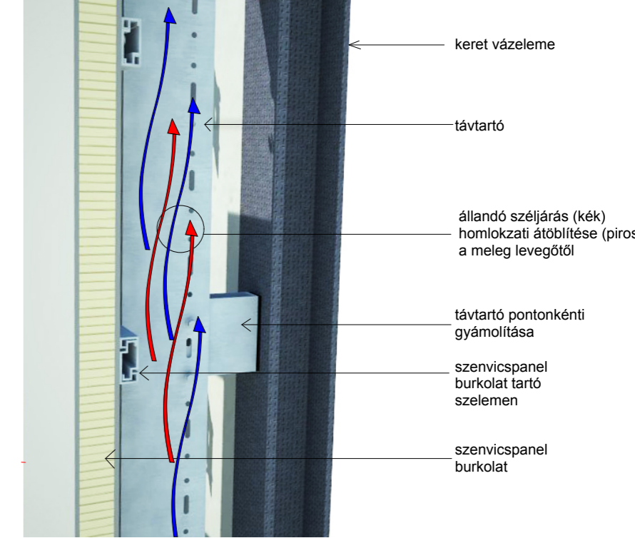
Részlet: szendvicspanel burkolat, szellőztető légszűrővel
