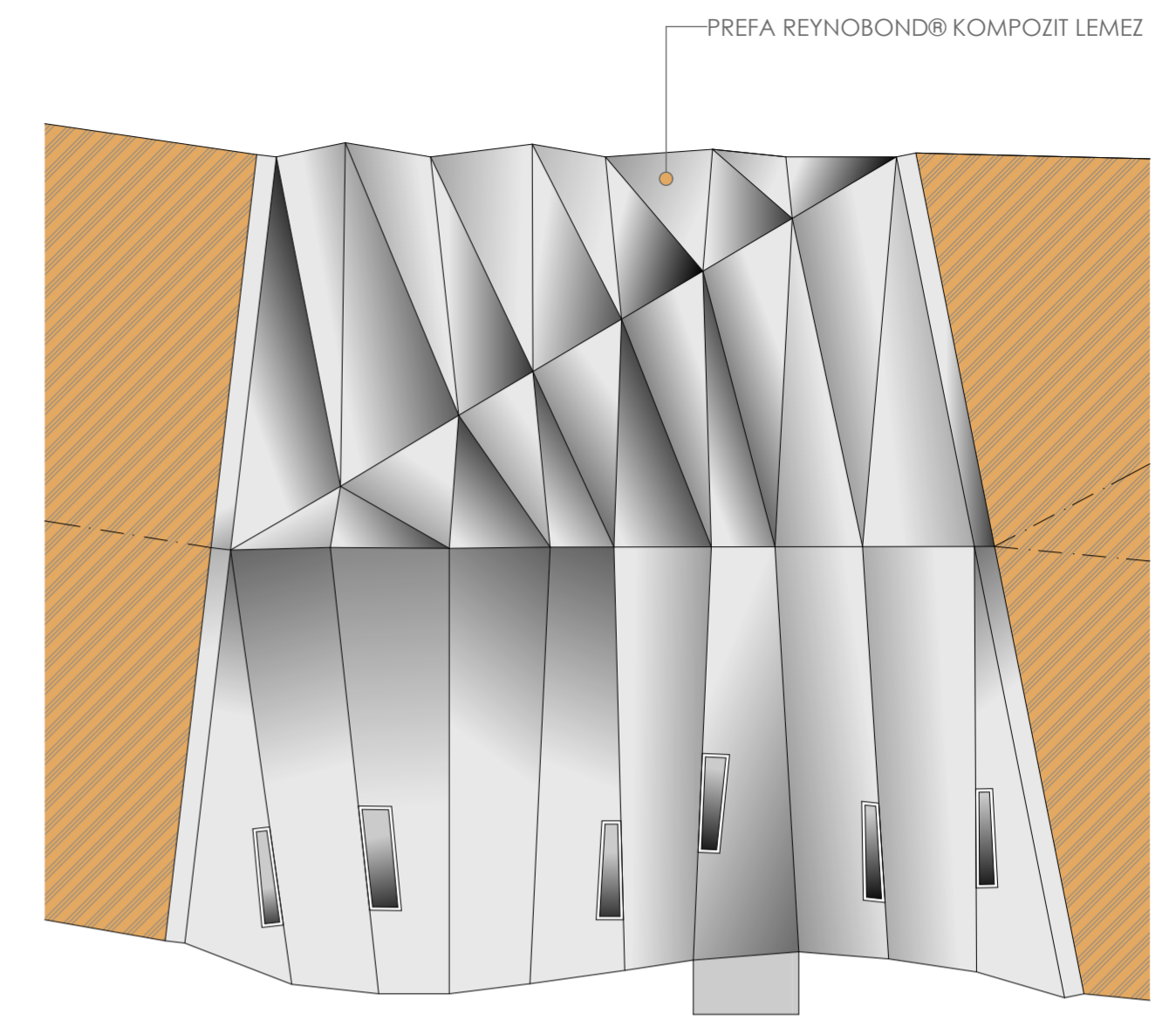
TETŐFELÜLNÉZETI ALAPRAJZ M 1:100
