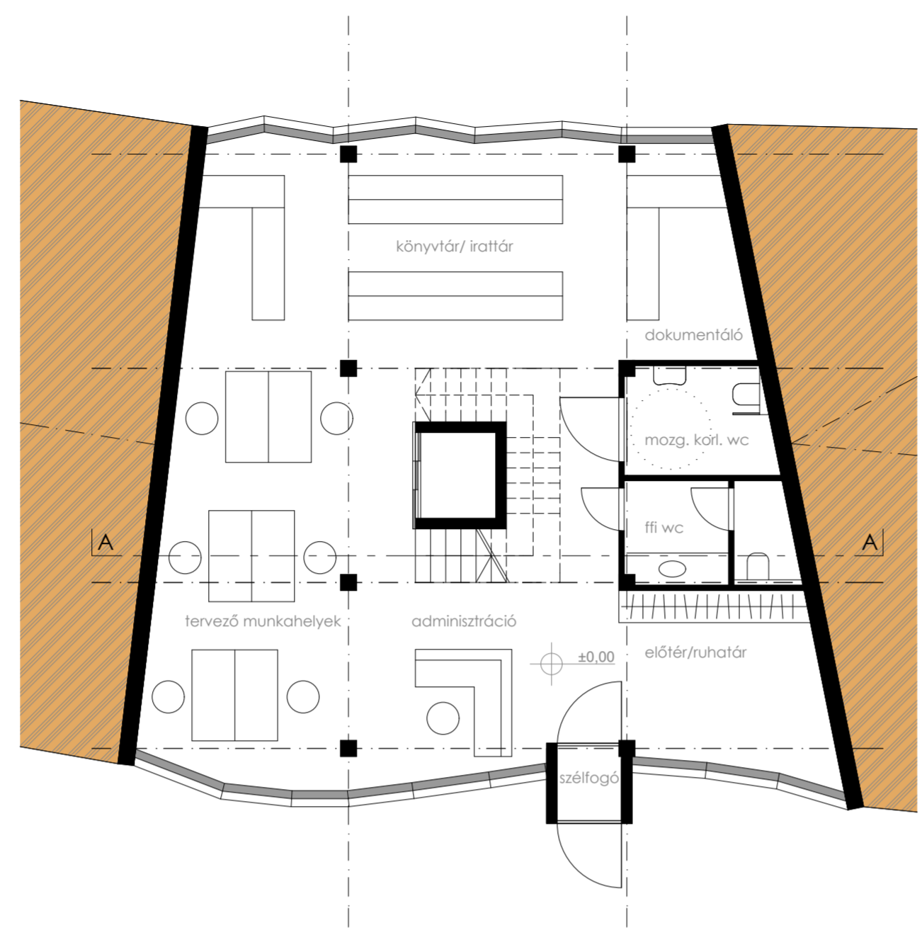
FÖLDSZINTI ALAPRAJZ M 1:100
