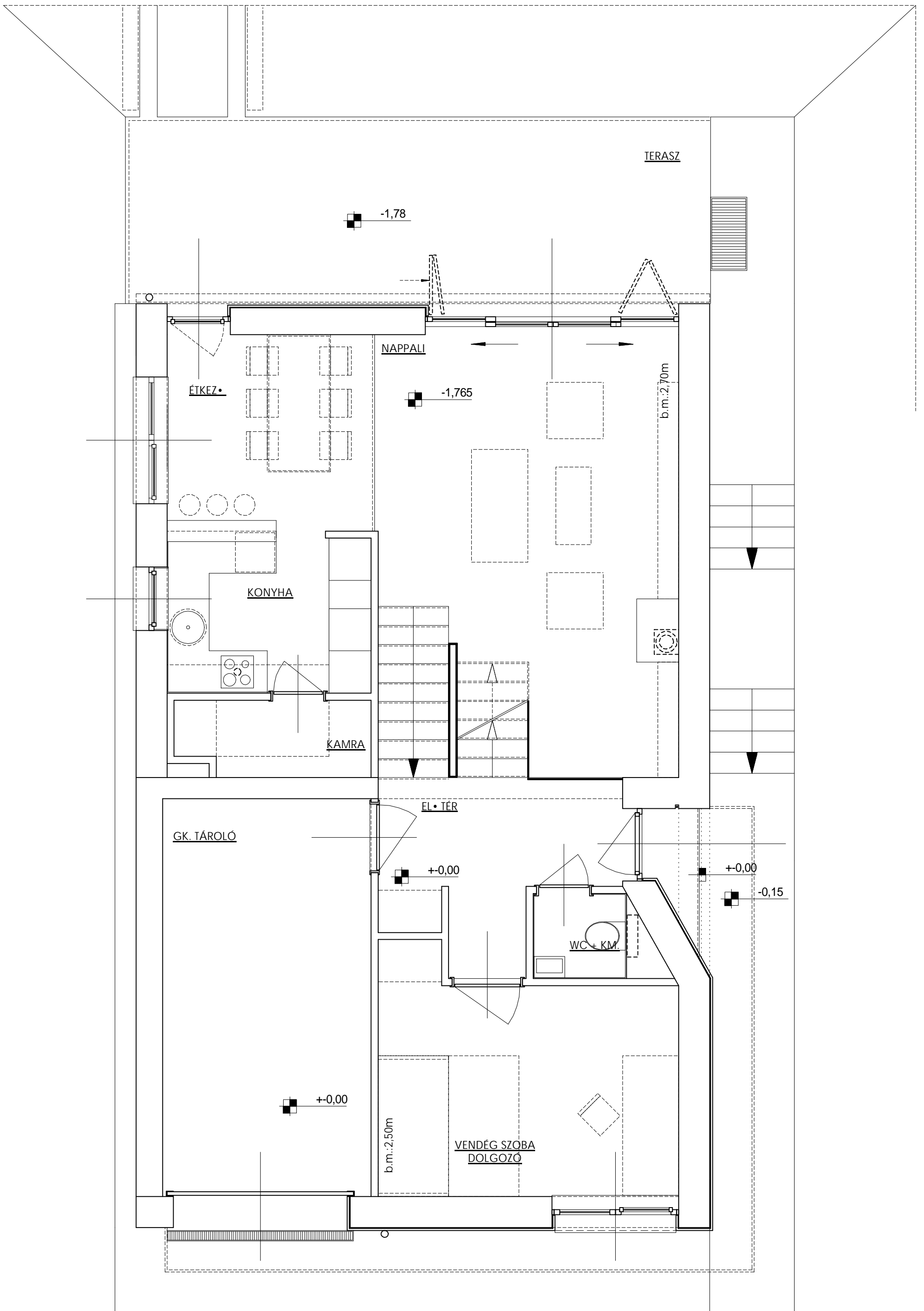
földszinti alaprajz
