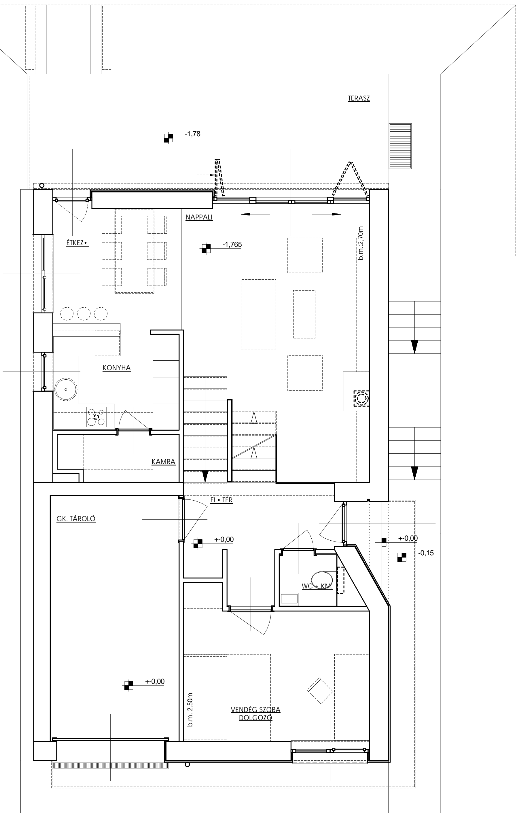
földszinti alaprajz
