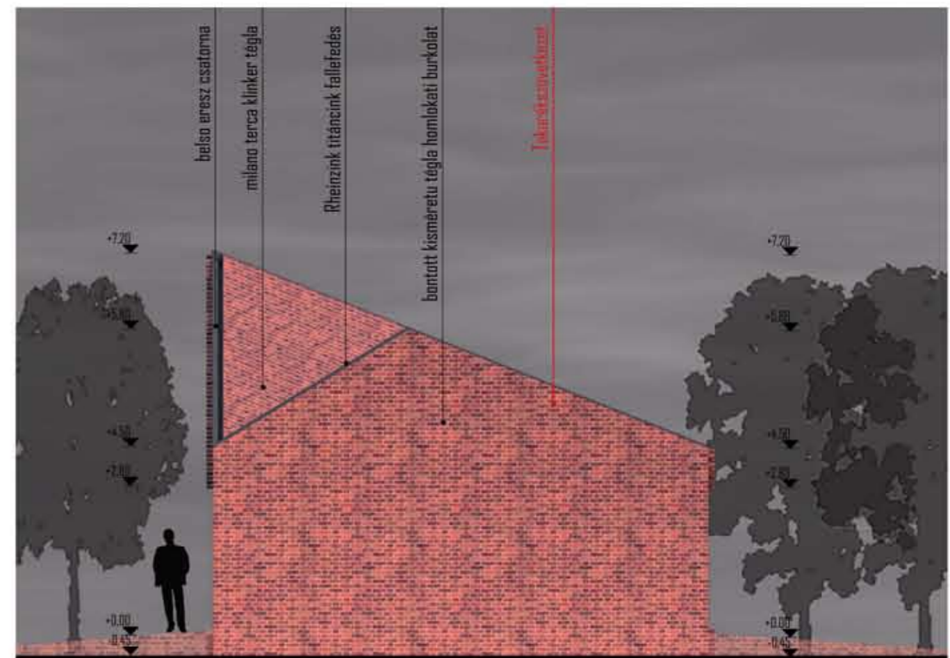
Észak-Nyugati homlokzat
