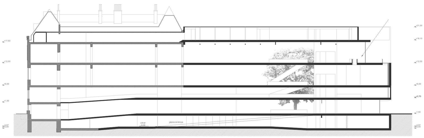
L-L METSZET 1:200
