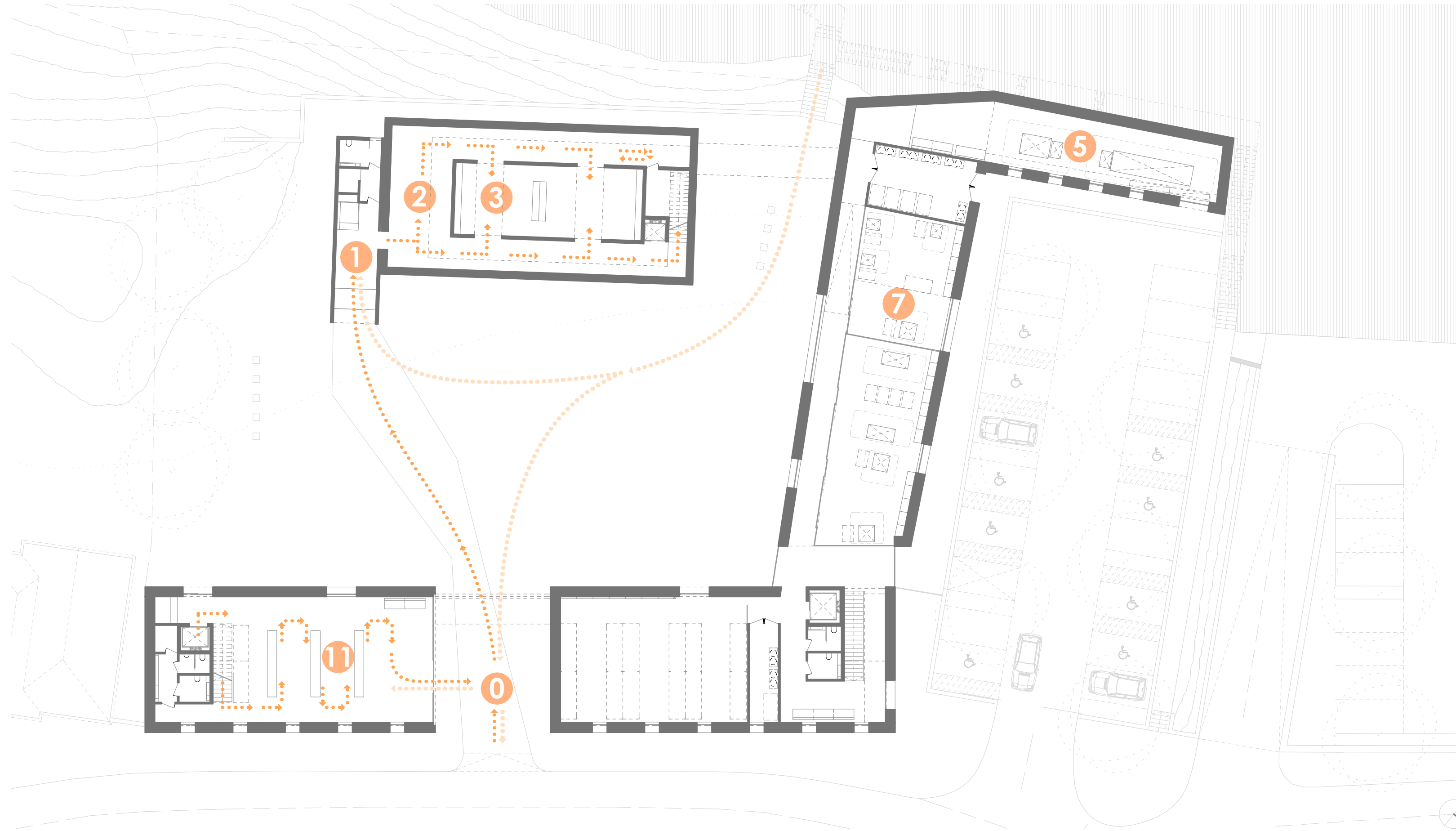
Az épület bejárása - földszinti alaprajz M 1:250
