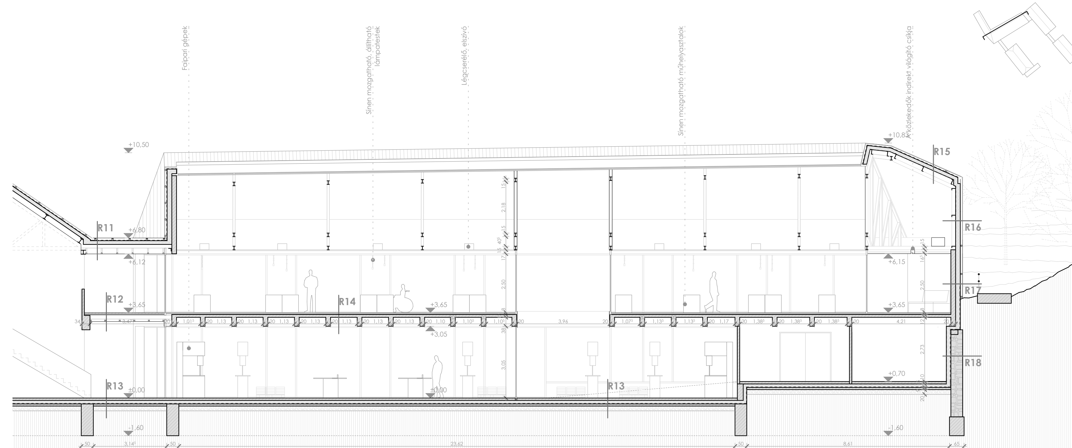
H-H metszet M 1:100
