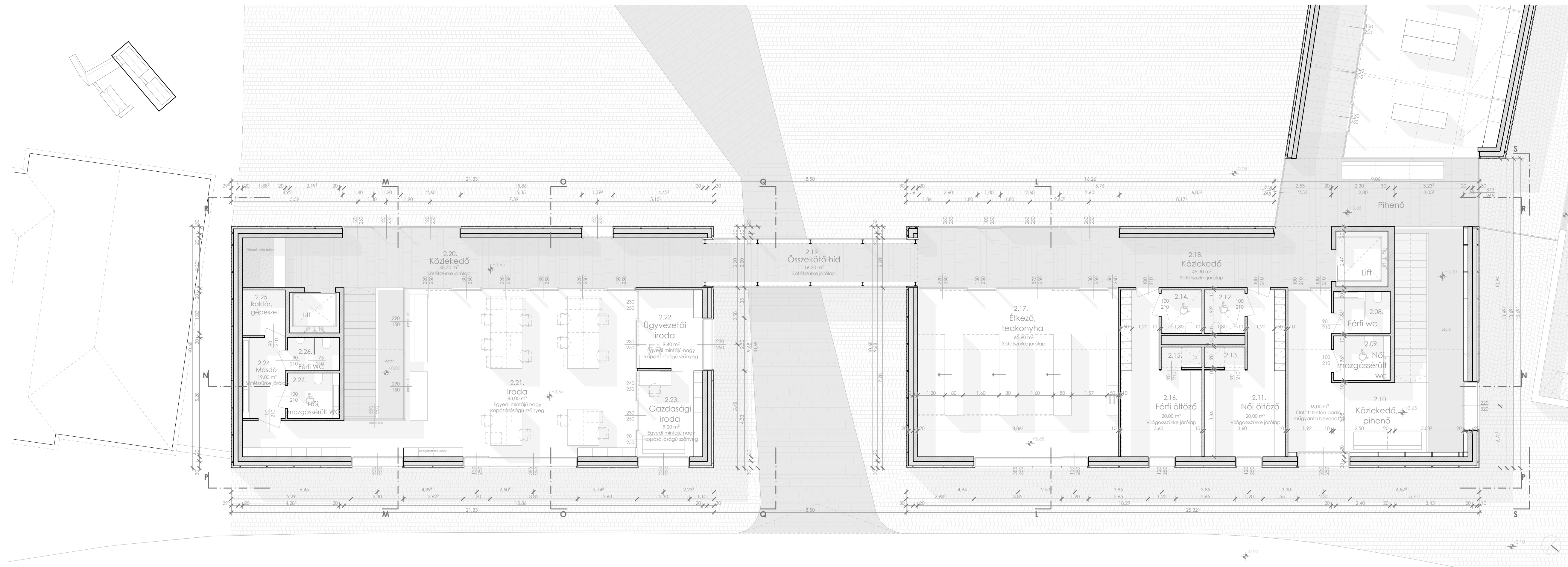
Emeleti alaprajzi részlet M 1:100
