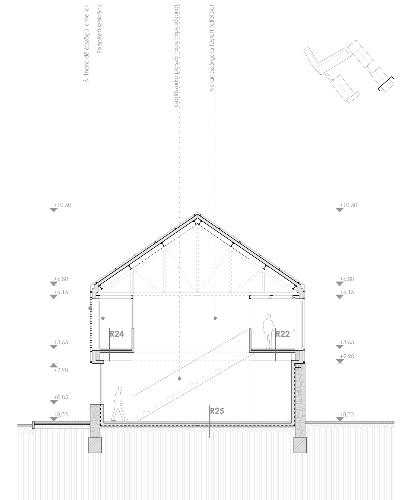
M-M metszet M 1:100
