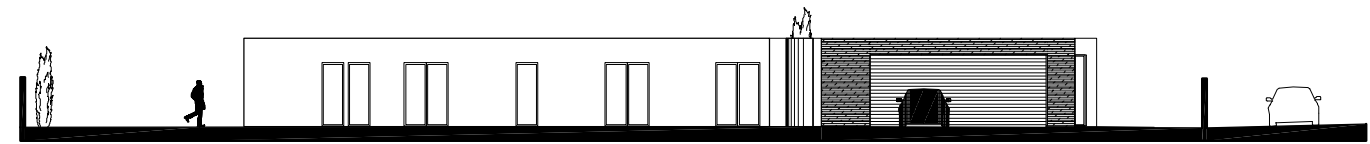
\\ALÇADO NASCENTE _ EAST ELEVATION
