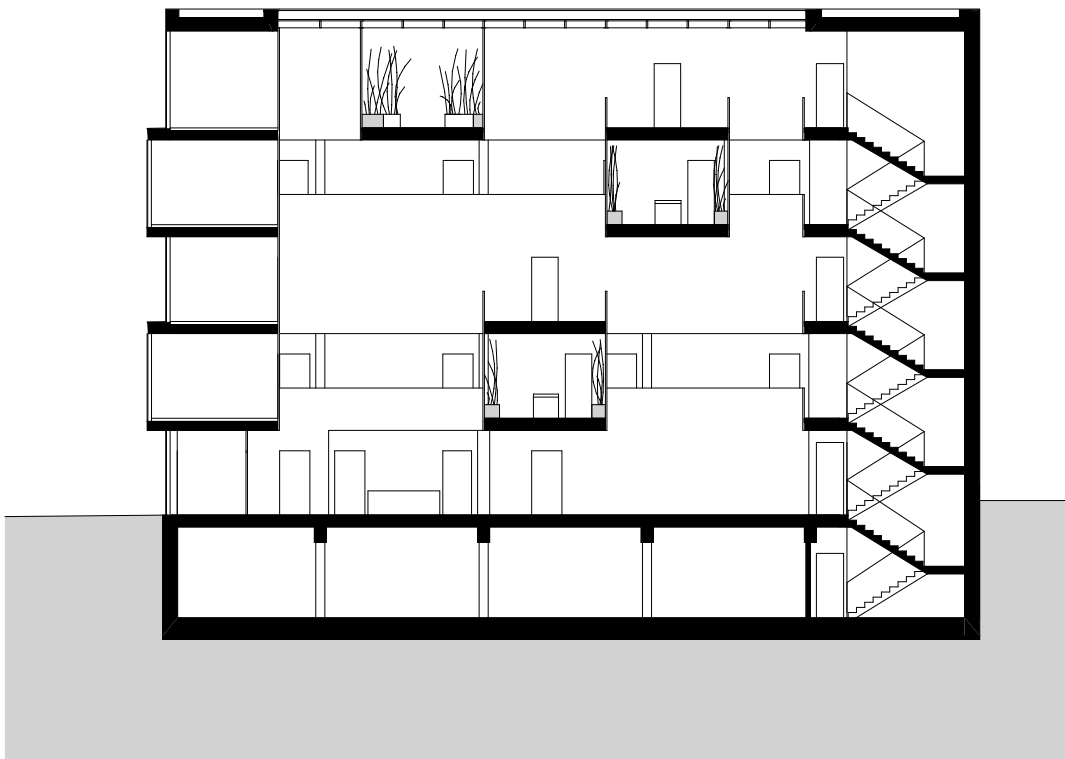
Geometria irodaház, Medve utca hosszmetszet
