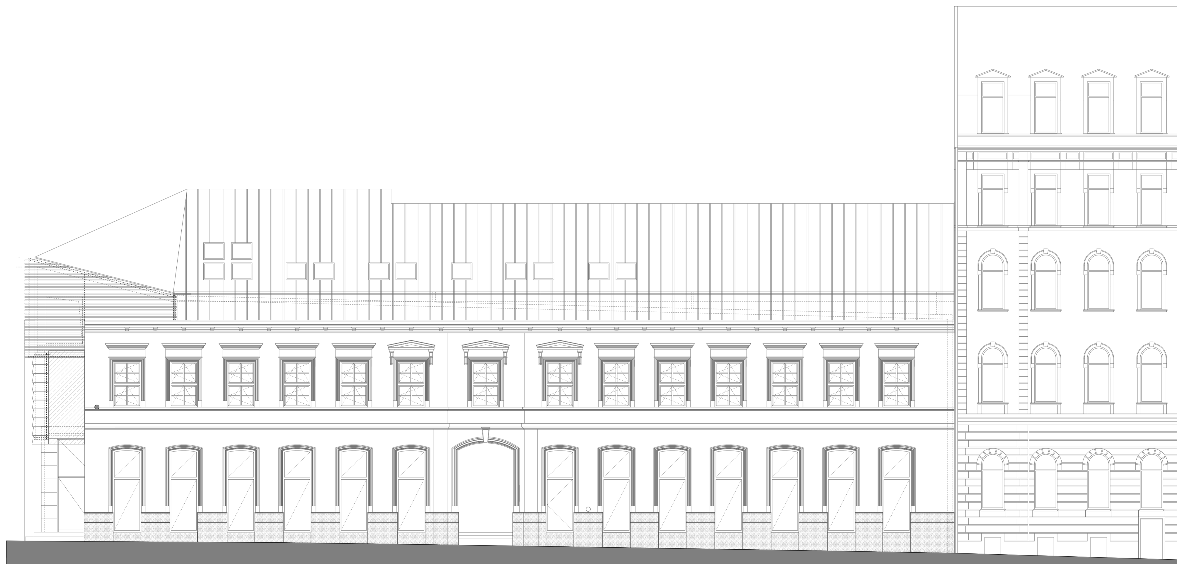
MÁTYÁS UTCAI HOMLOKZAT
