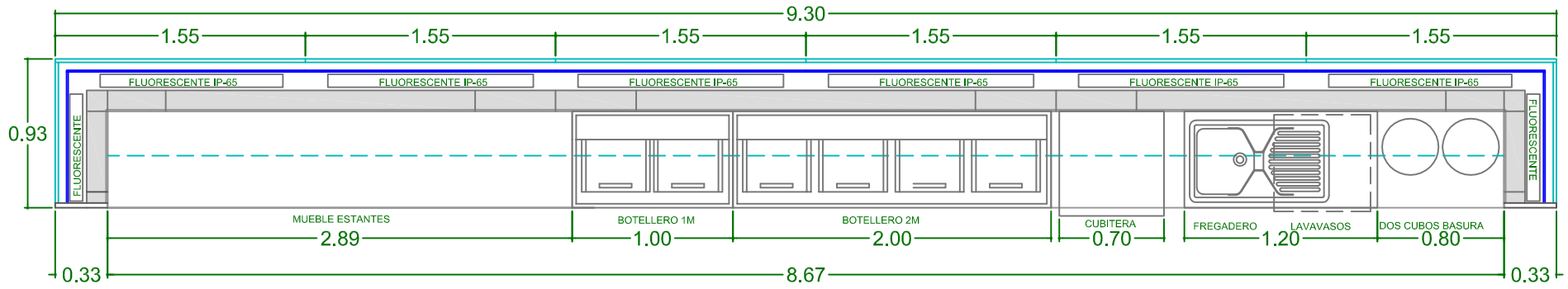
Planta de la barra del bar
