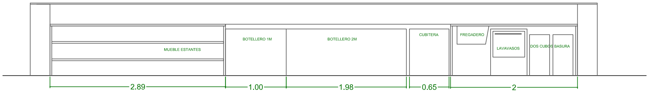
Alzado interior de la barra del bar
