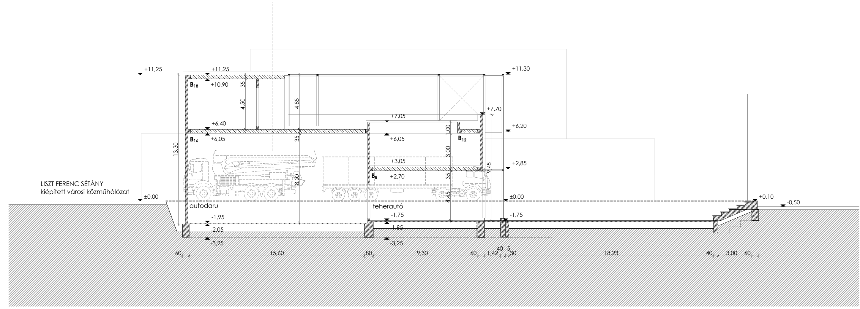
SZERKEZETÉPÍTÉS ORGANIZÁCIÓS HELYSZÍNRAJZ ÉS METSZET M=1:200
