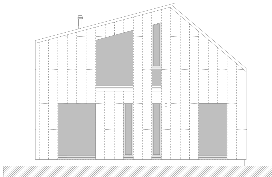
DÉLI HOMLOKZAT
