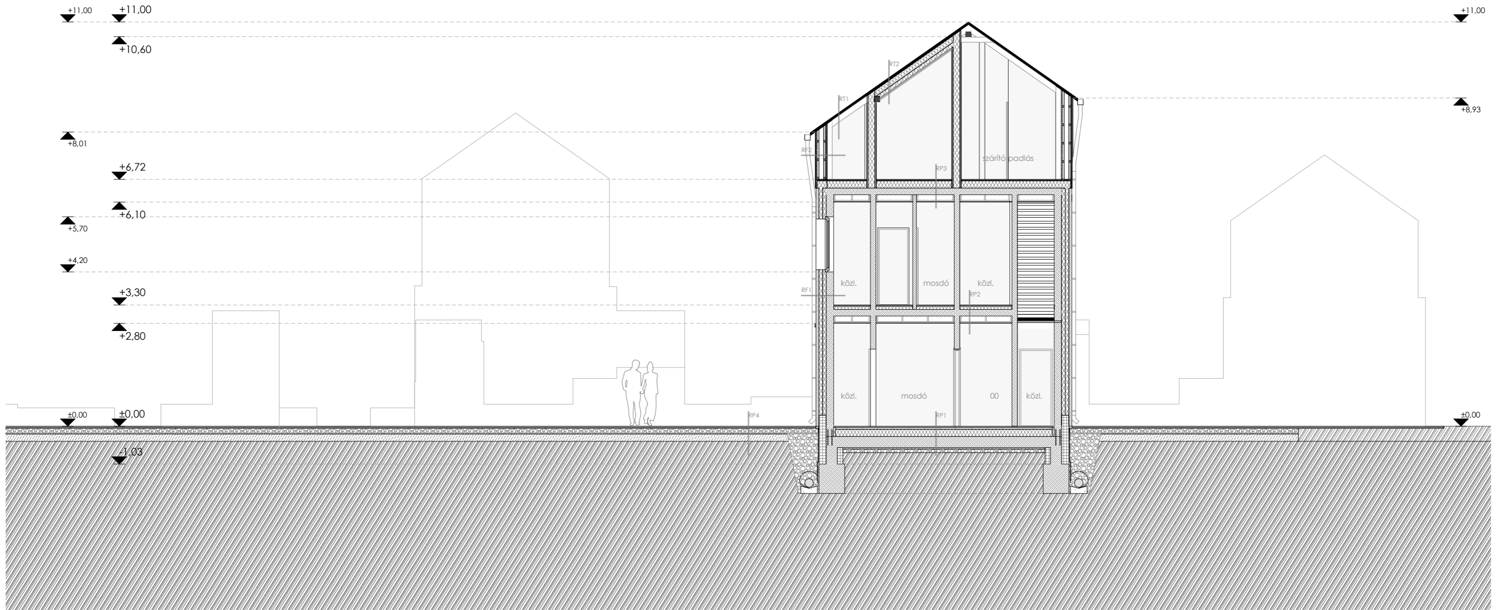
1-1 metszet patika m 1:100
