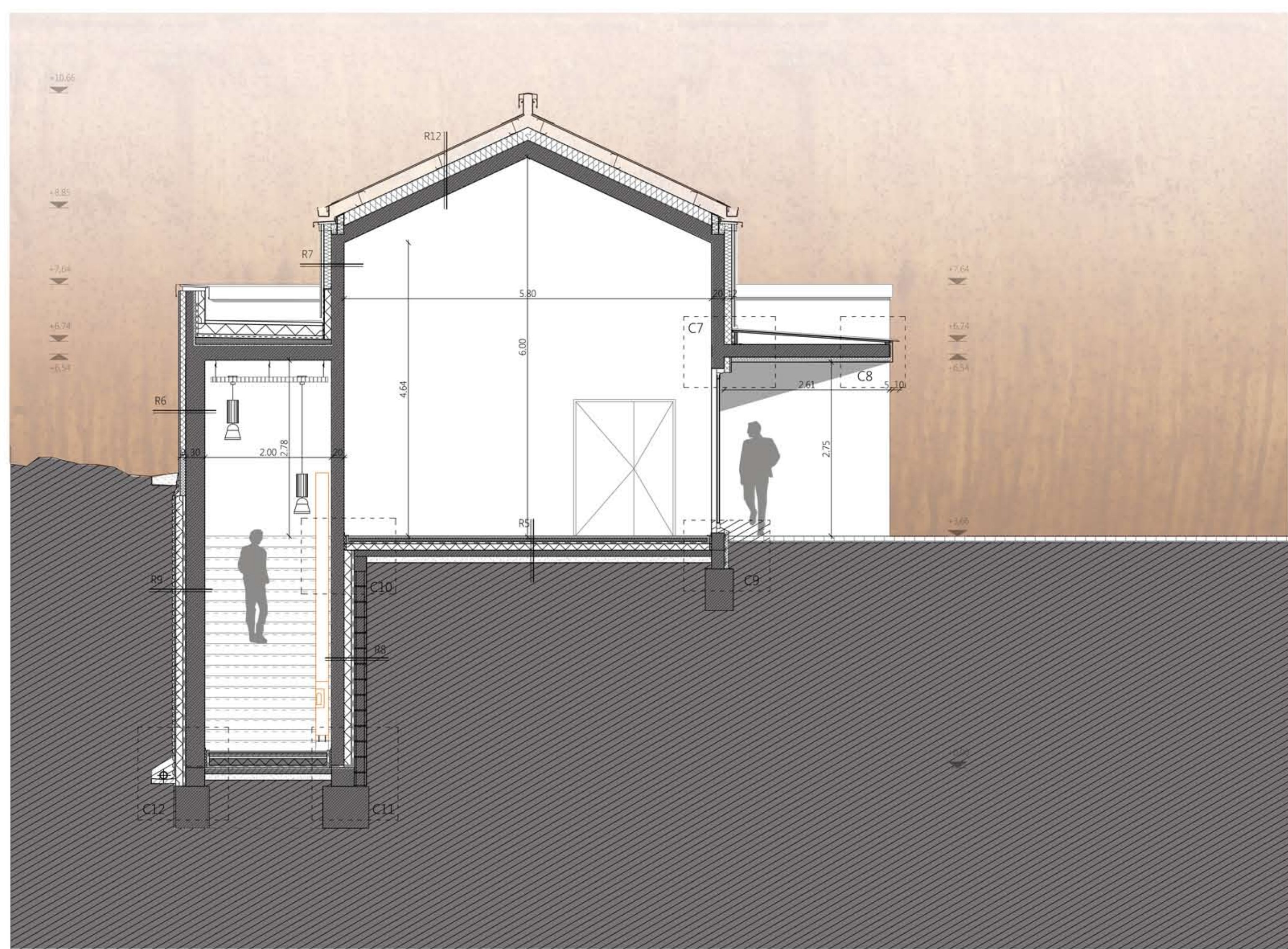
6 - 6 metszet - műhely
