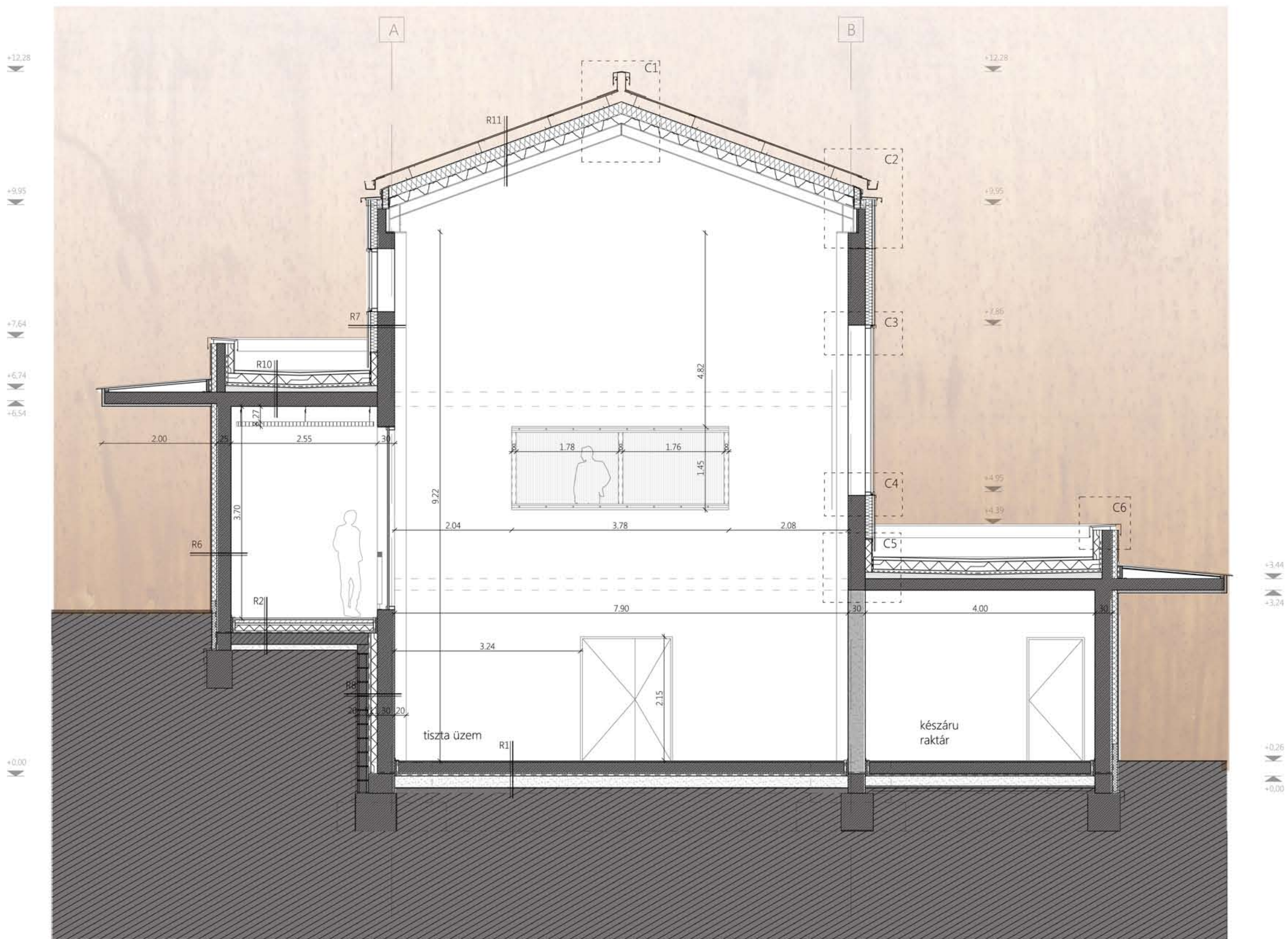
5 - 5 metszet - üzem
