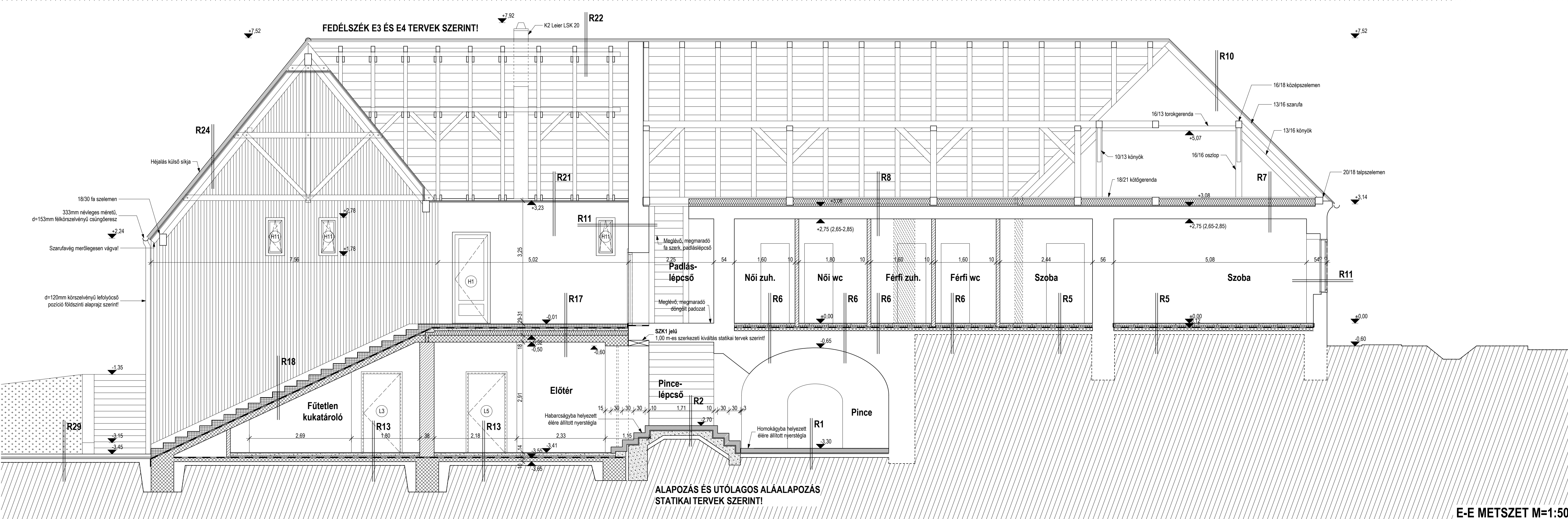
E-E METSZET M=1:50
