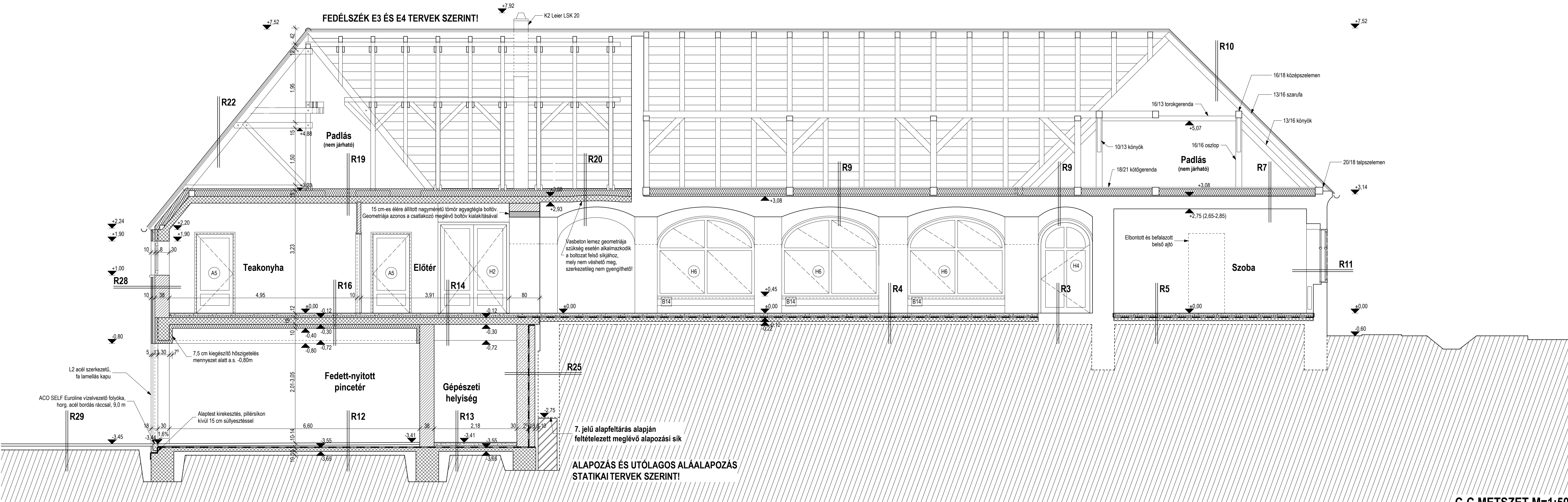
C-C METSZET M=1:50
