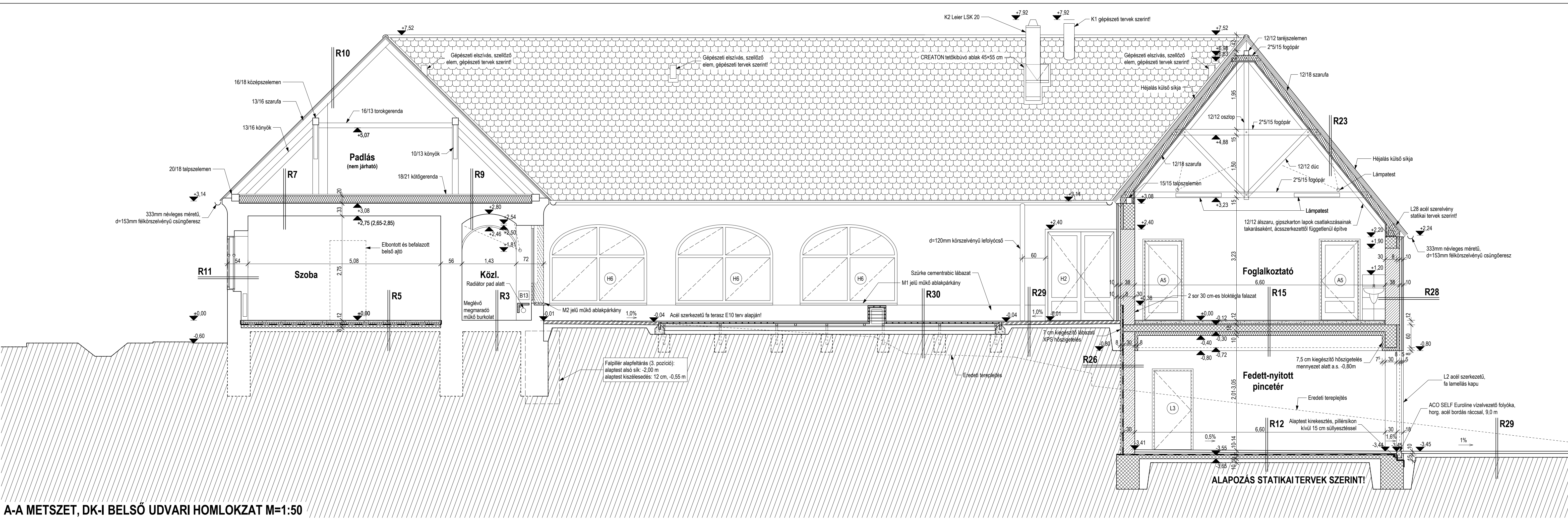
A-A METSZET, DK-I BELSŐ UDVARI HOMLOKZAT M=1:50
