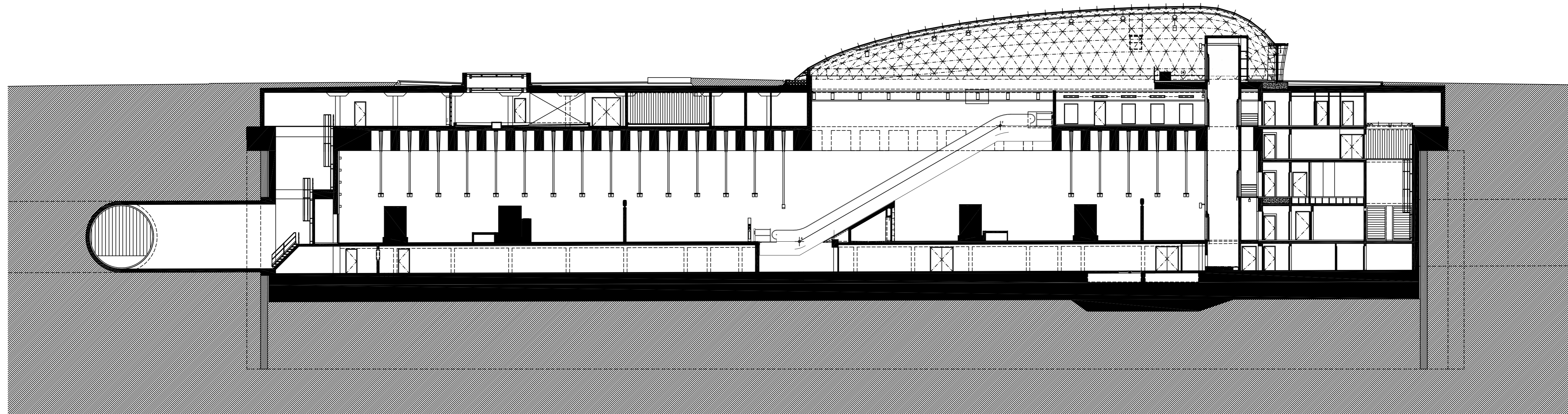
longitudinal section
