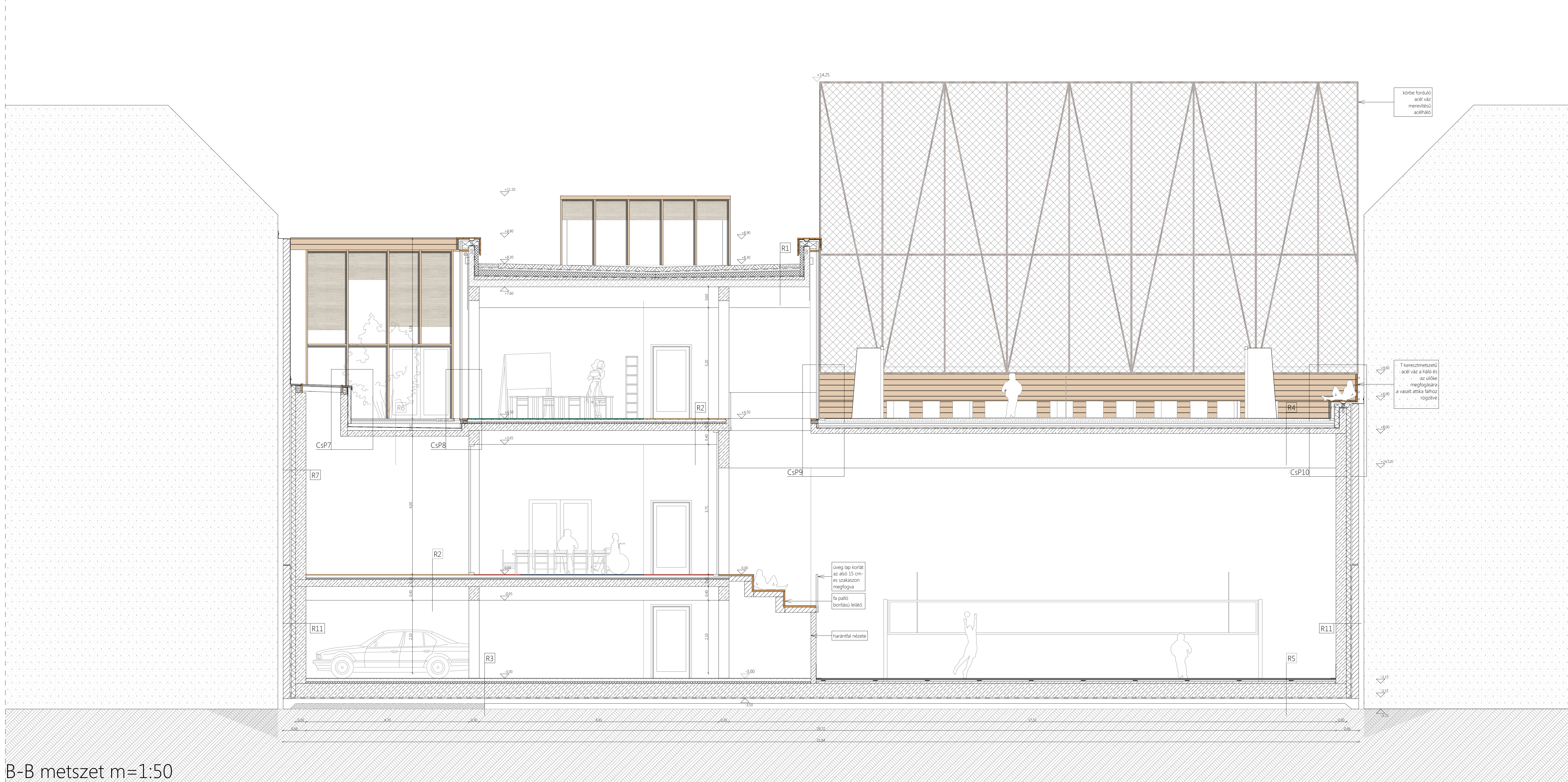
B-B metszet m=1:50
