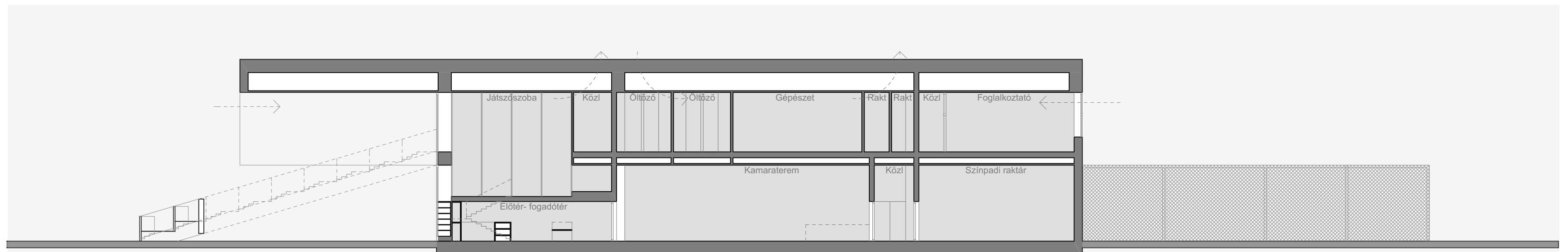
B-B METSZET M 1:200
