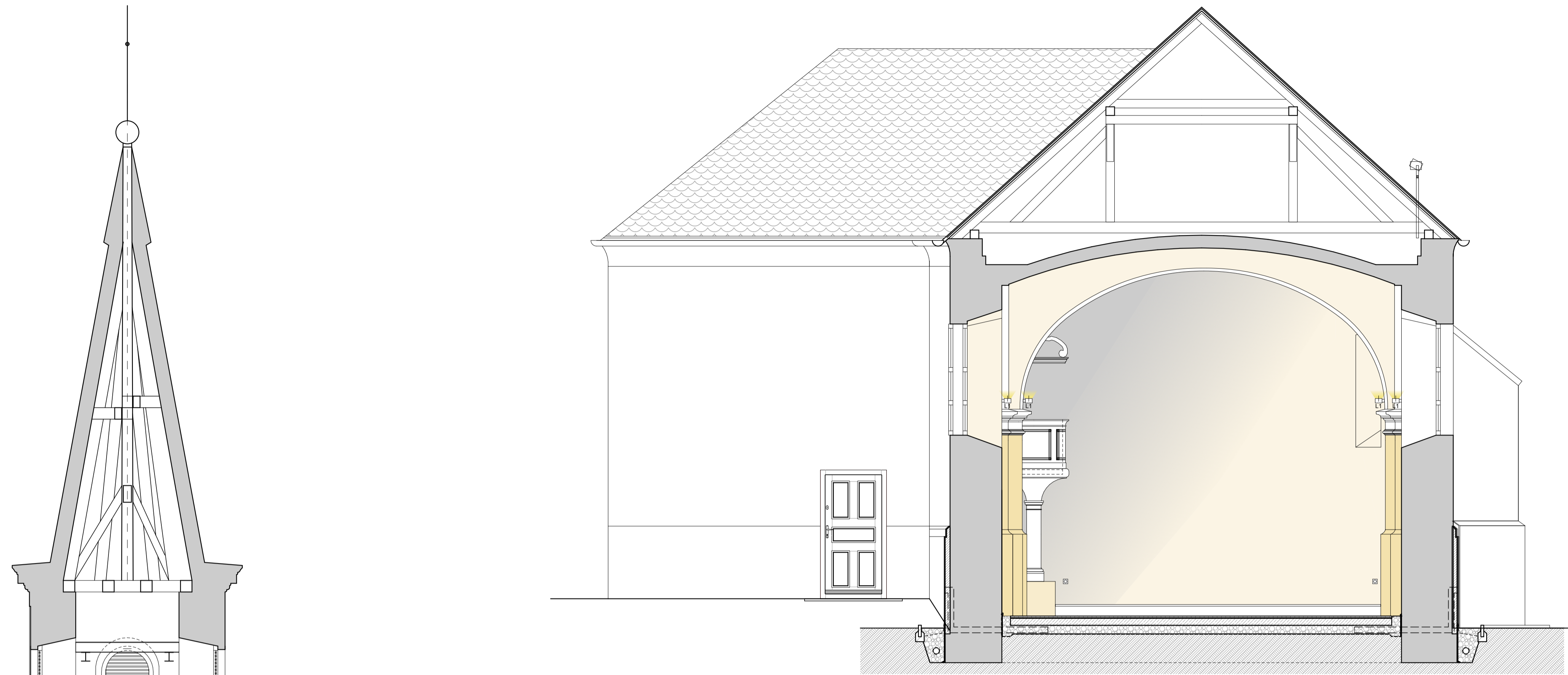
Tervezett B-B metszet M 1:50
