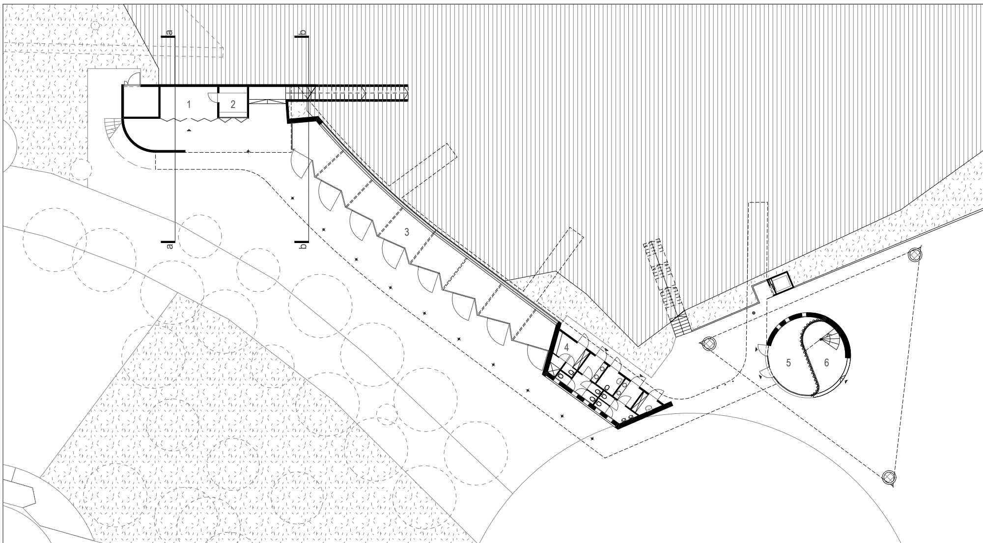
földszinti alaprajz
