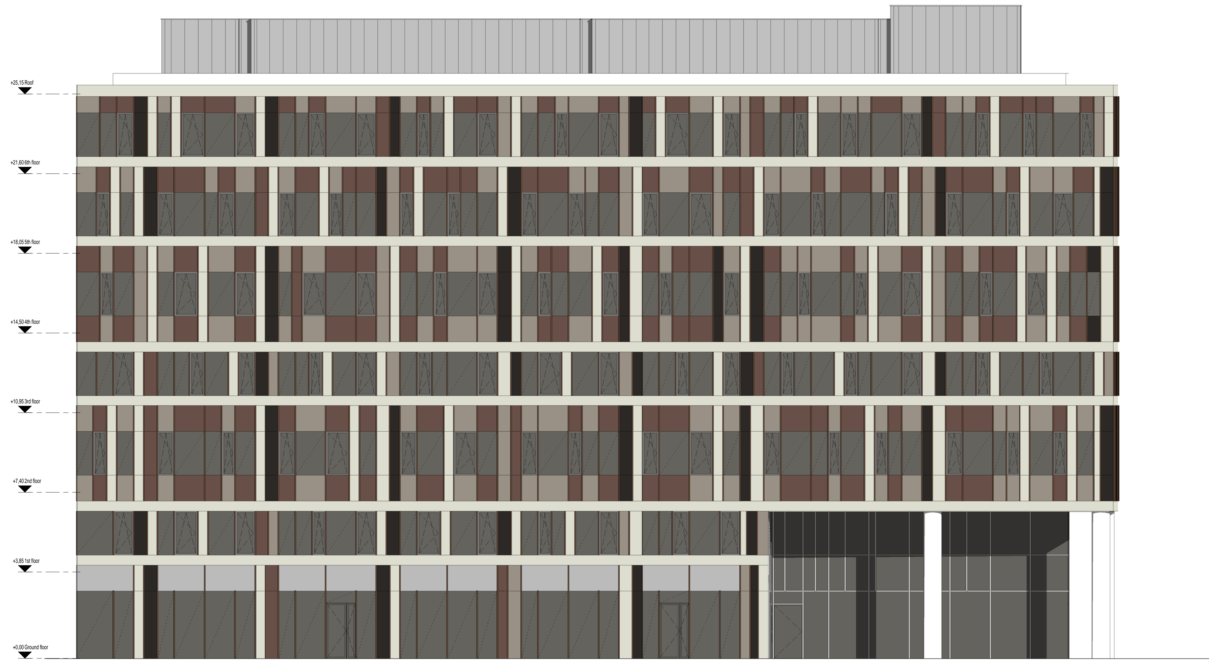
Bence utca Facade M I Scale 1 : 100
