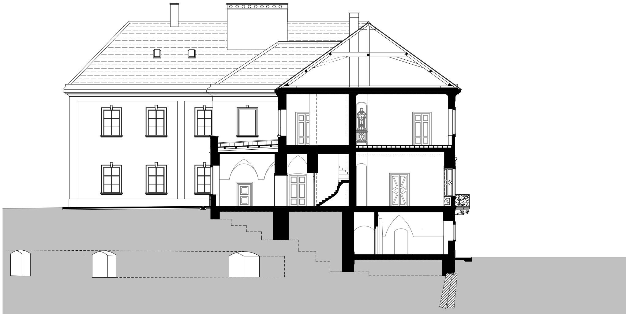
C-C metszet
