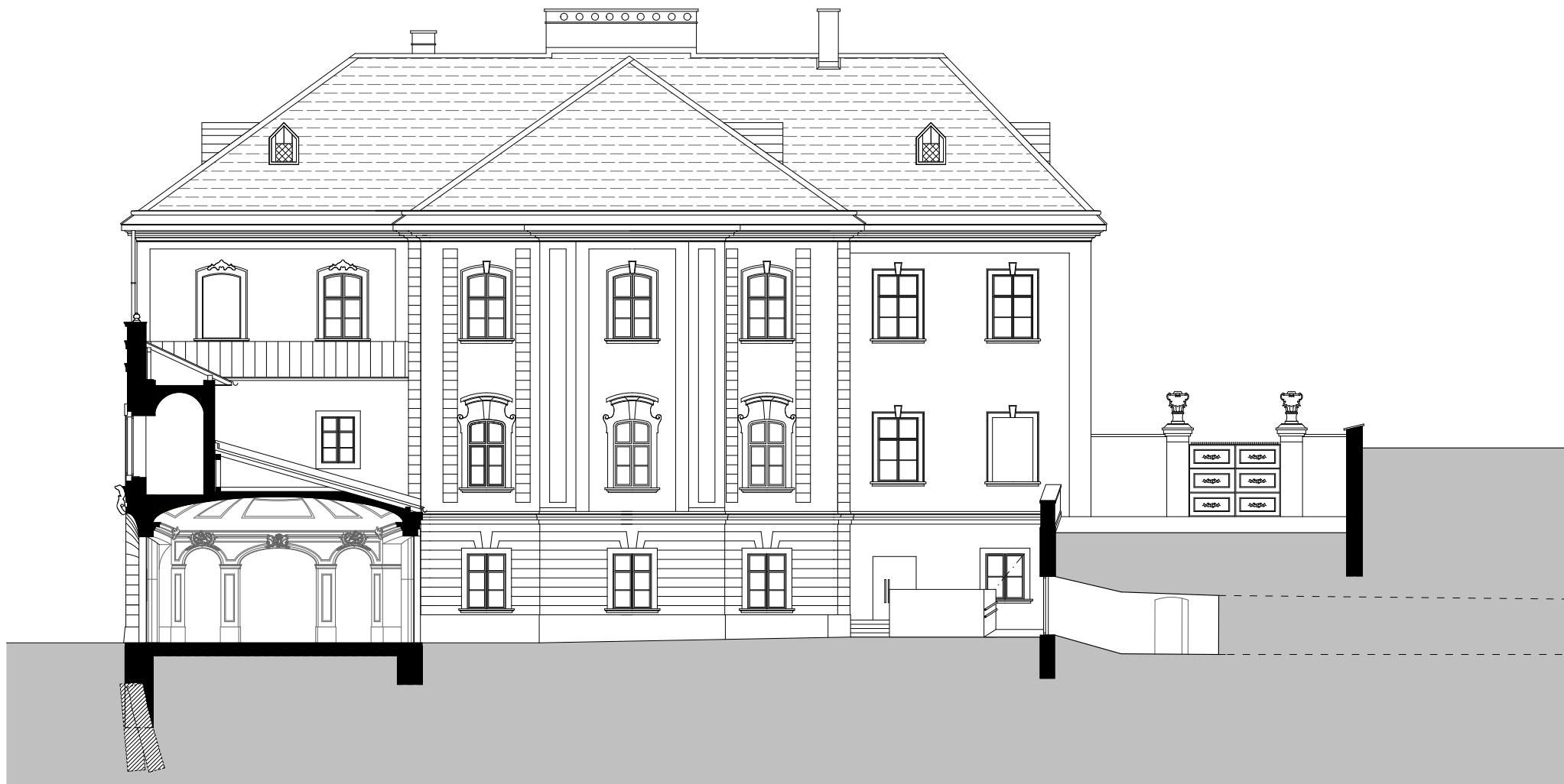
E-E metszet
