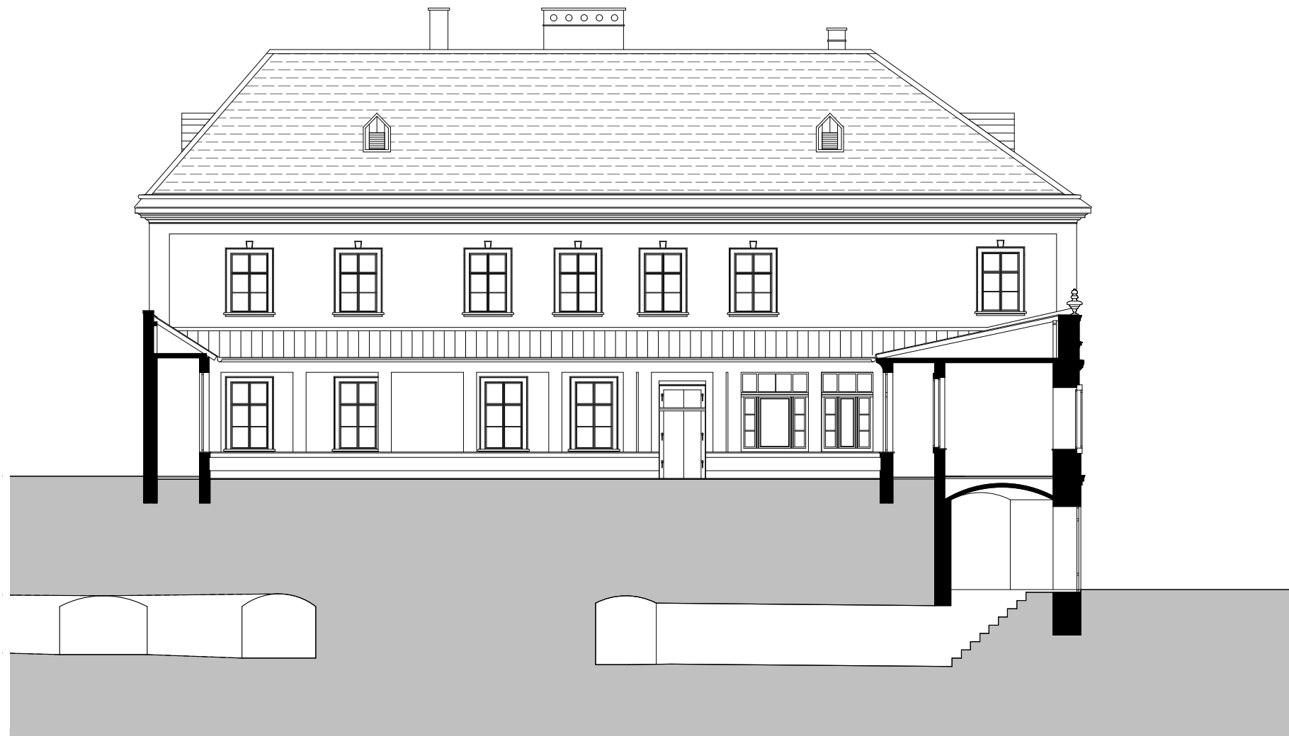
Délkeleti homlokzat
