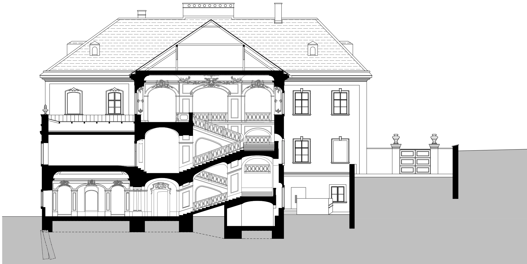
F-F metszet
