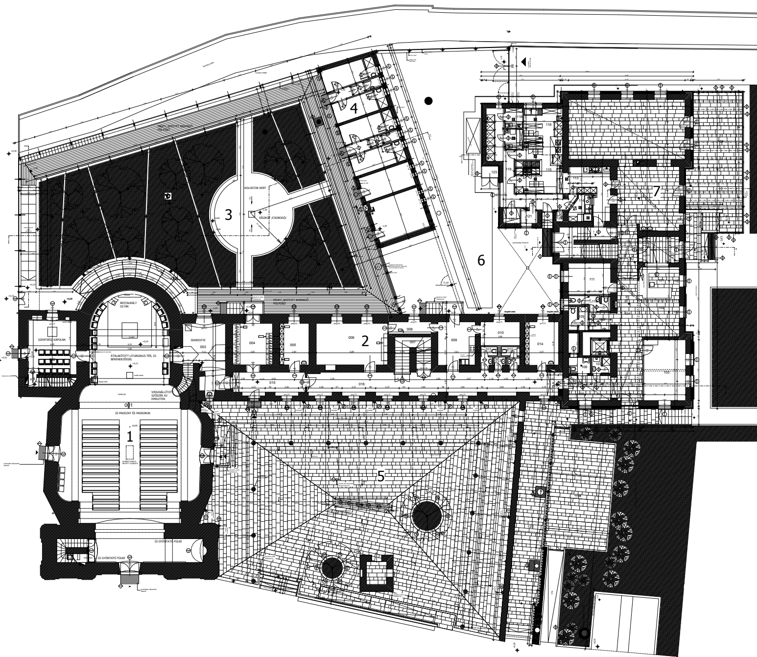
TEMPLOM, RENDHÁZ, ZARÁNDOKHÁZ ALAPRAJZA
