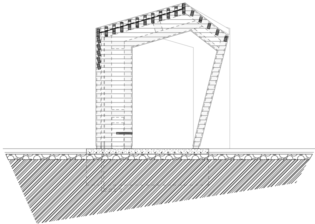
a-a metszet
