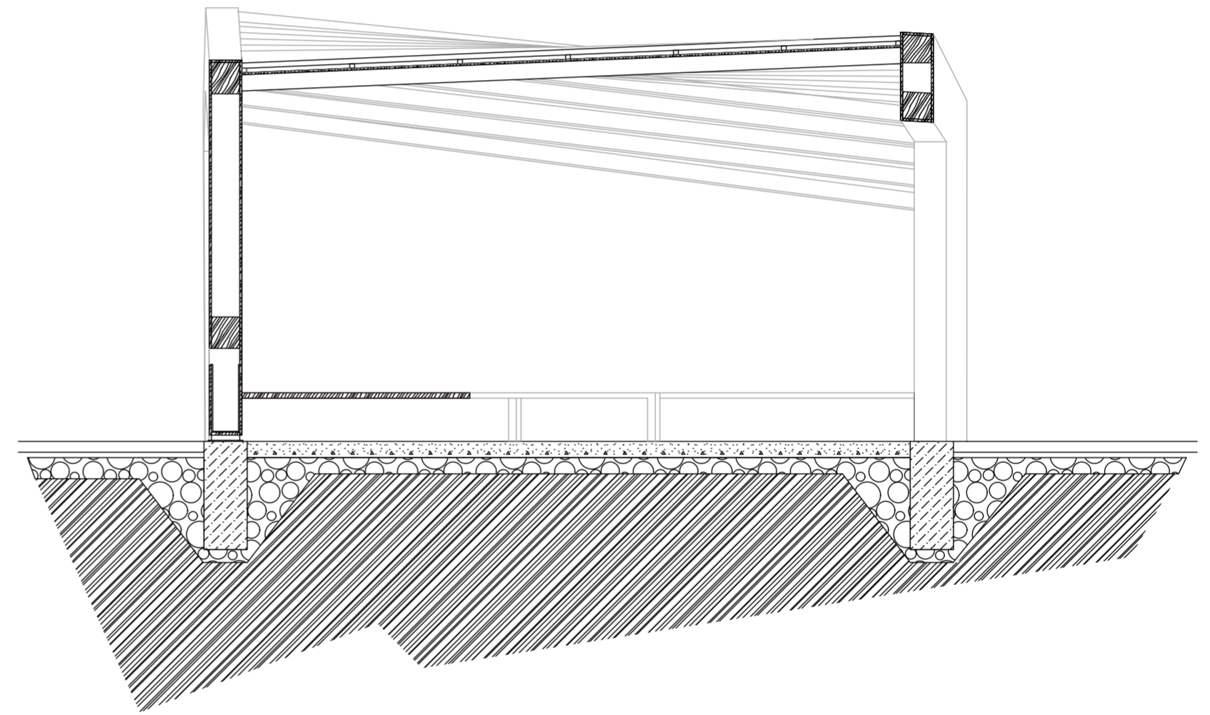
b-b metszet
