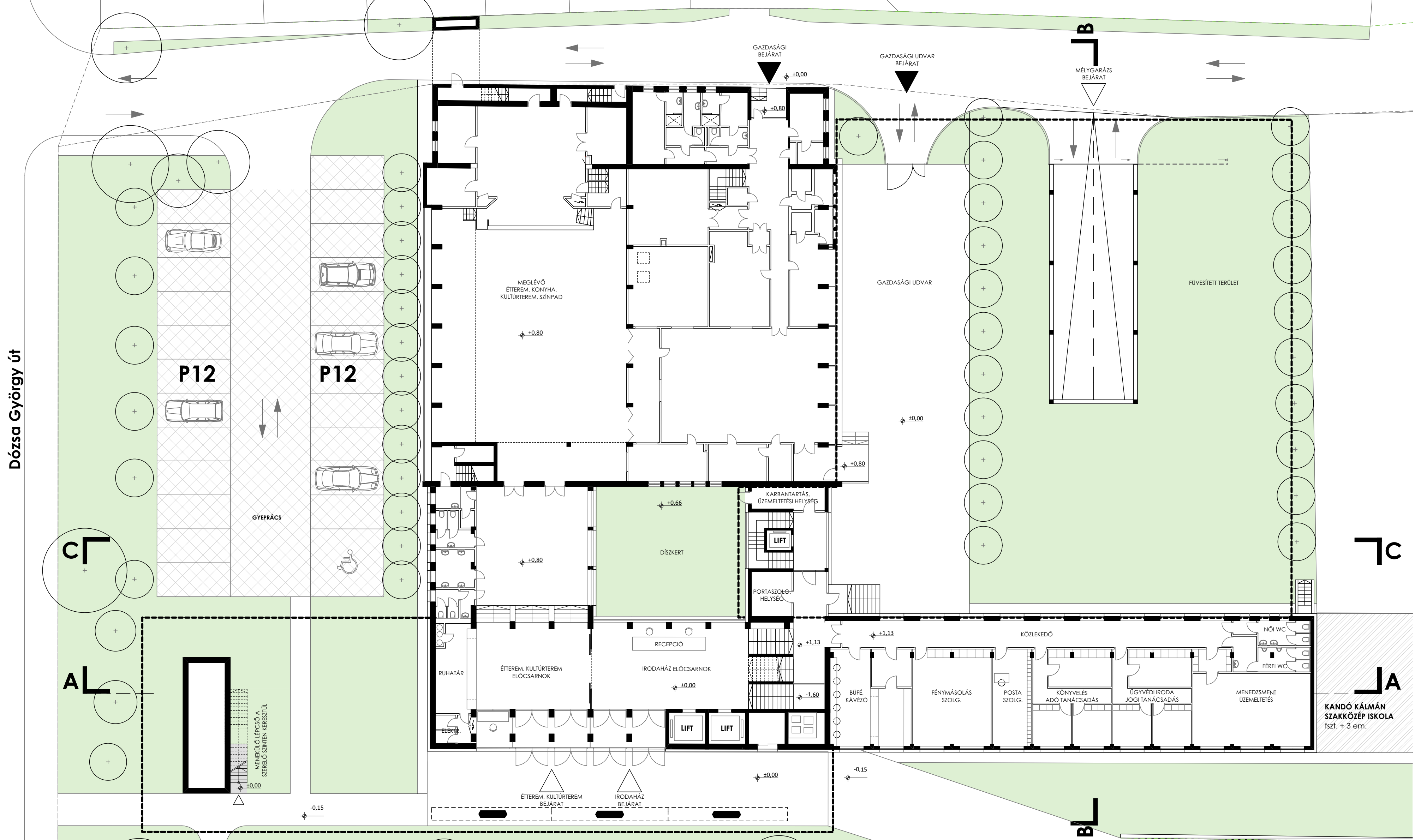
FÖLDSZINTI ALAPRAJZ | M=1:200
