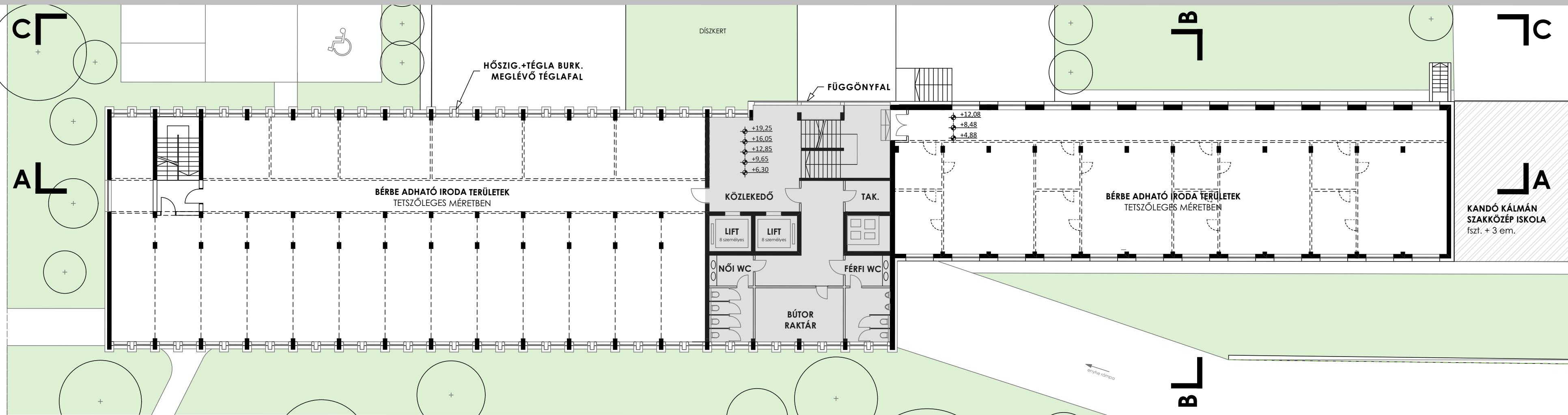
ÁLTALÁNOS EMELETI ALAPRAJZ | M=1:200
