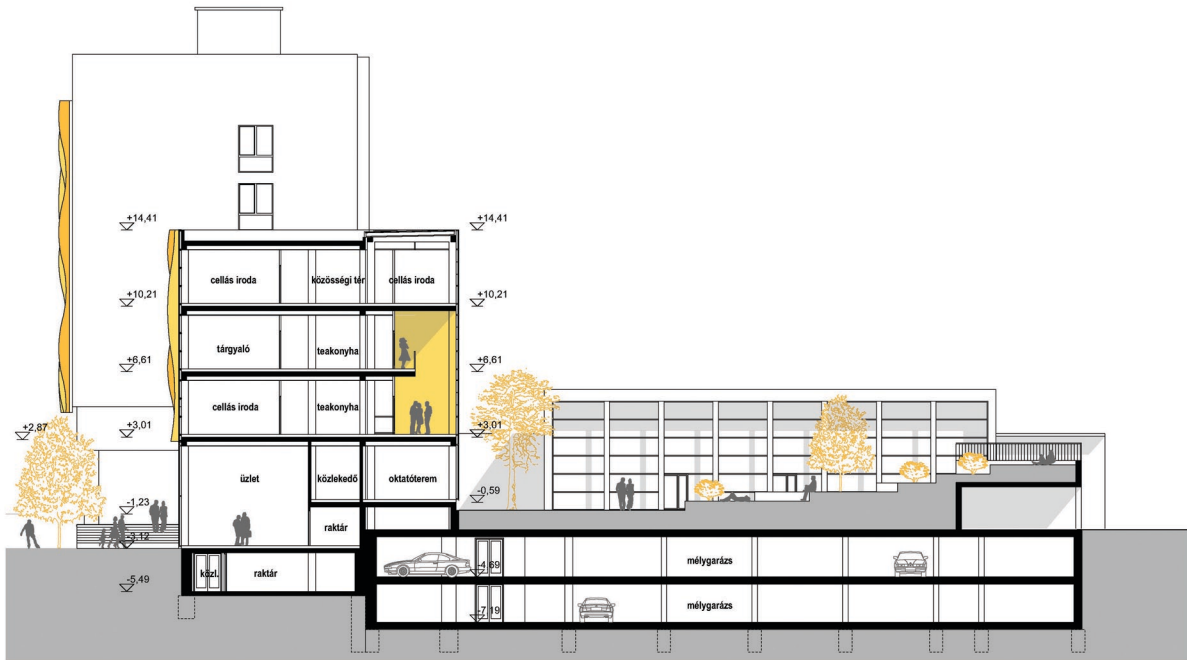
3-3 metszet és Keleti homlokzat
