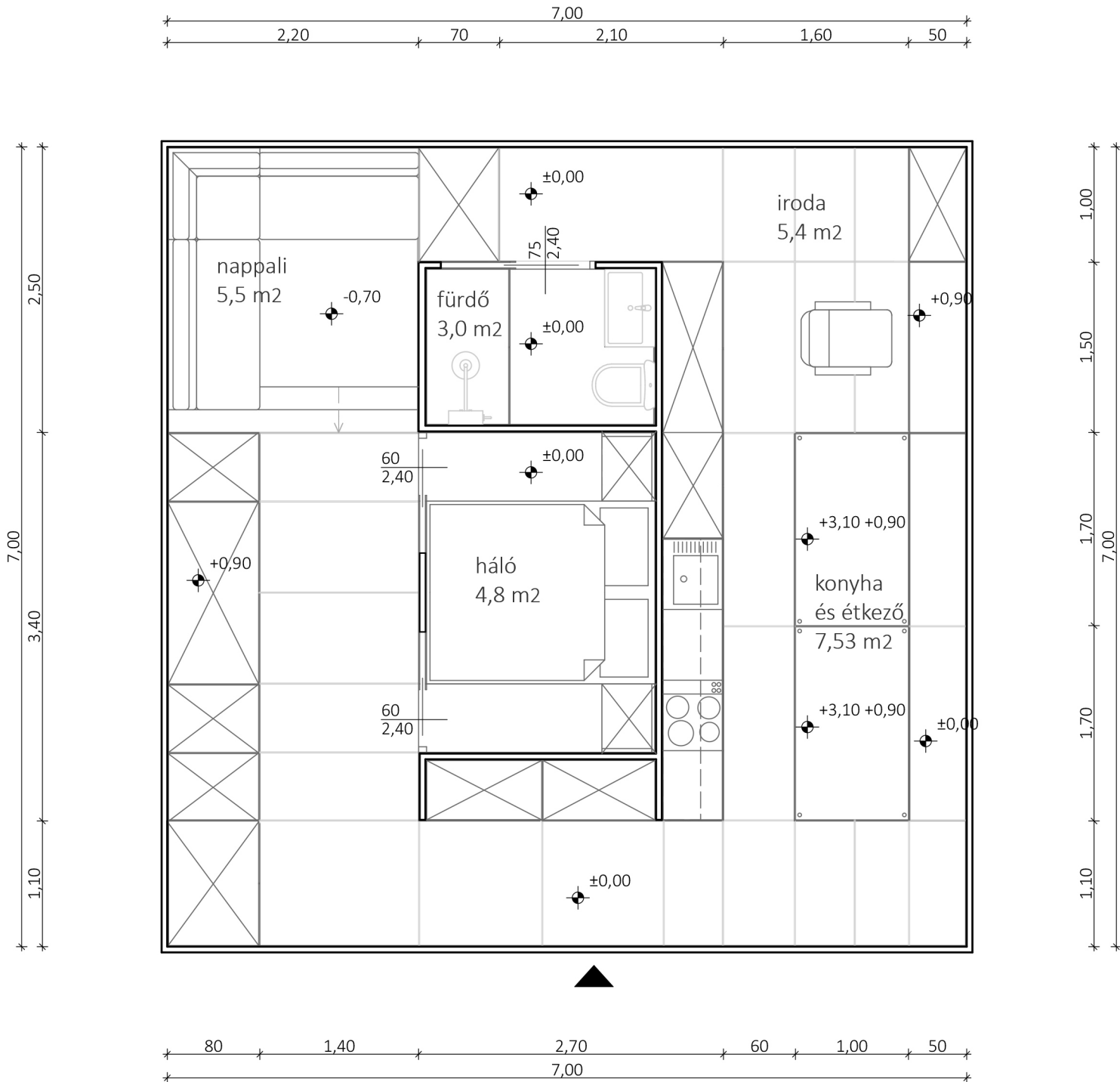
Alaprajz - nyitott állapot M1:50
