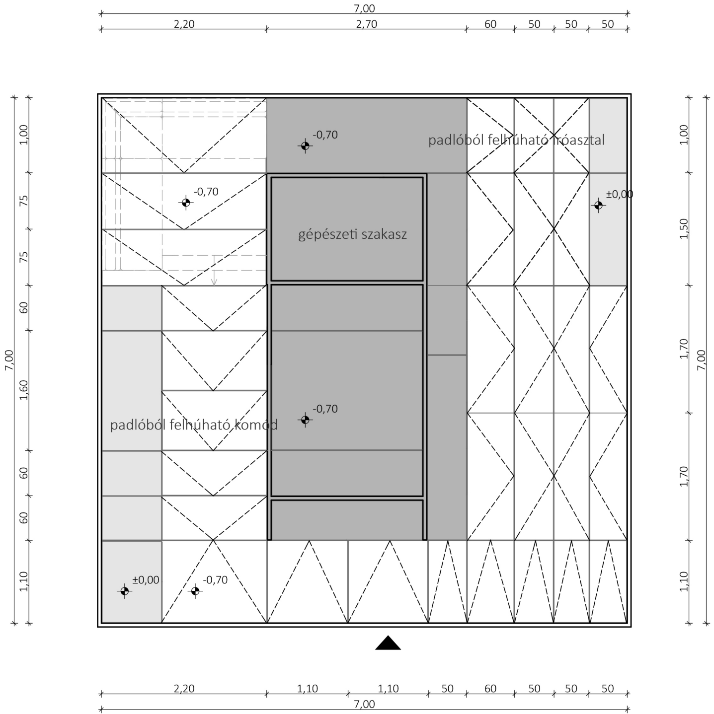
Alaprajz - padló tárolók M1:50
