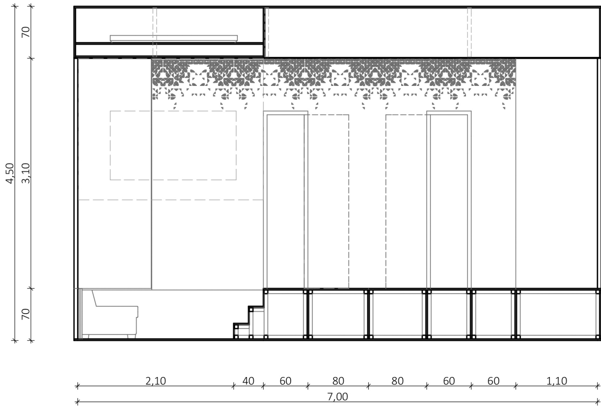
Falnézet és burkolatkiosztás M1:50
