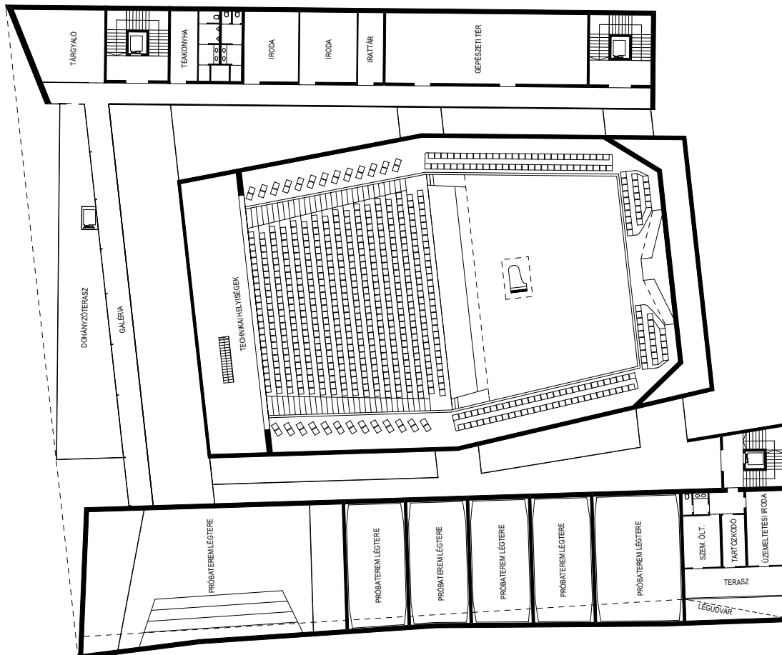
KOMOLYZENEI KONCERTTEREM - III. EMELET
