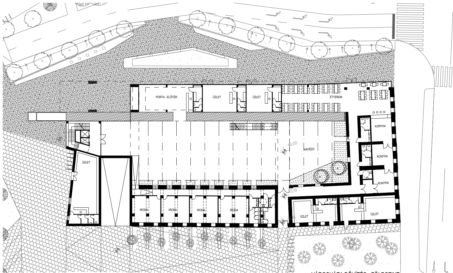
VÁROSHÁZA BŐVÍTÉS - FÖLDSZINT
