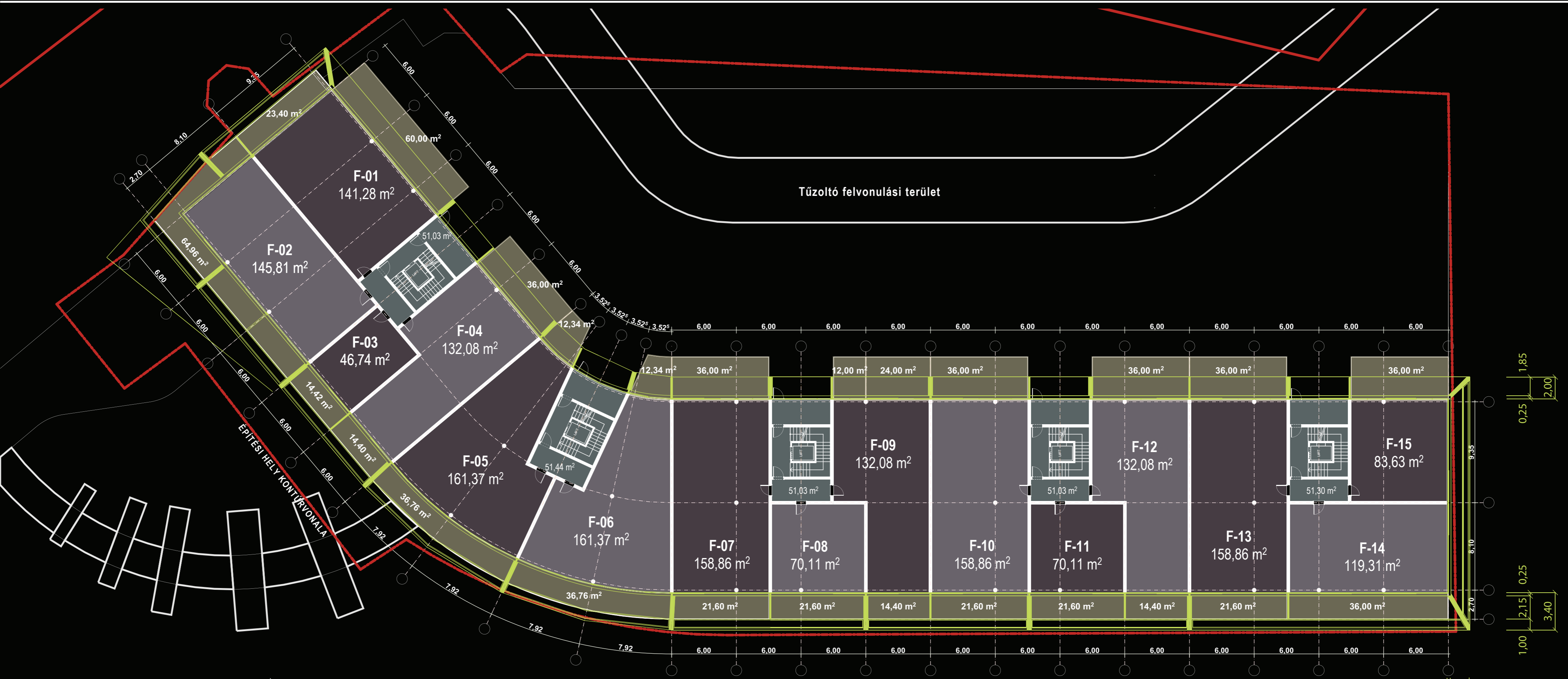
Földszinti alaprajz M = 1 : 250
